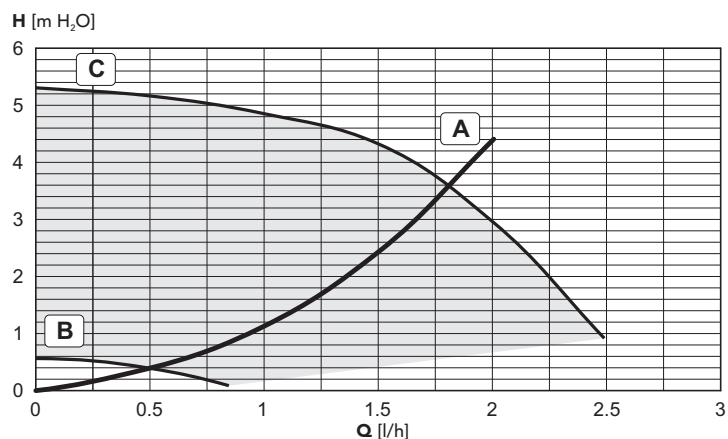
рис. 28 - Потери нагрузки/напор циркуляционного насоса iXinox 25 K 50
