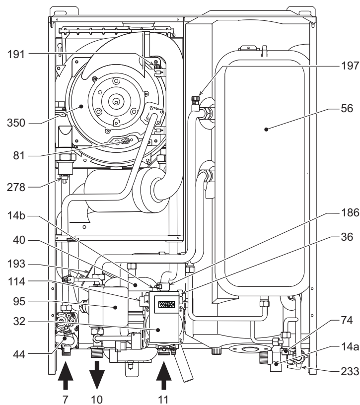
fig. 27 - Vista frontale
