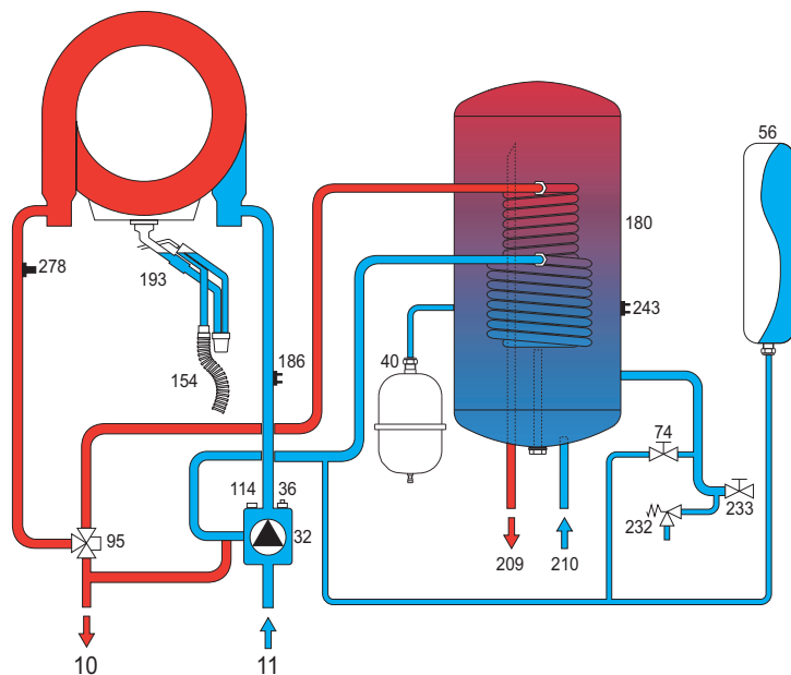
fig. 28 - Circuito idraulico
