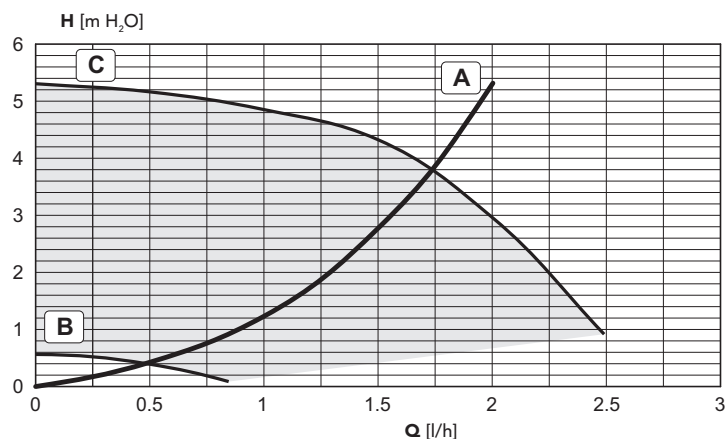
рис. 29 - Потери нагрузки/напор циркуляционного насоса iXinox 32 K 50
