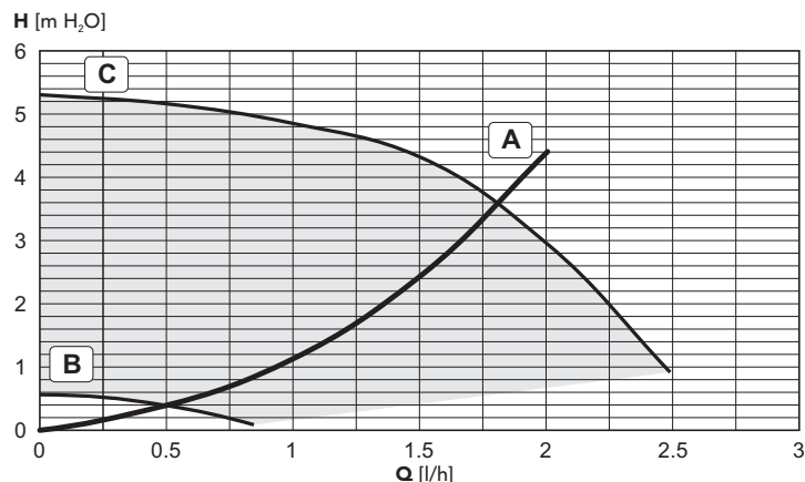
fig. 29 - Perdite di carico / prevalenza circolatore iXinox 25 K 50
