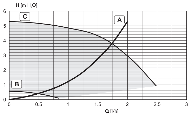
fig. 30 - Perdite di carico / prevalenza circolatore iXinox 32 K 50
