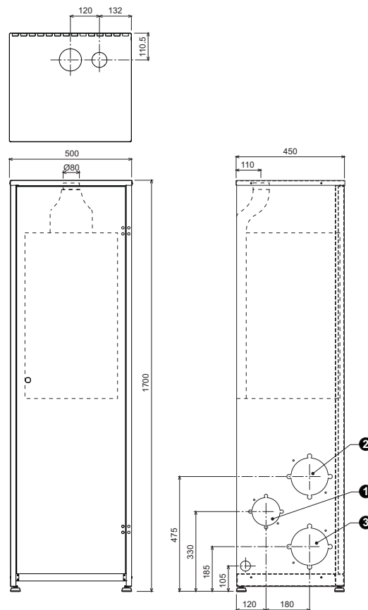
fig. 61 - Dimensioni e attacchi modello FUTURIA POWER 80 - 125
