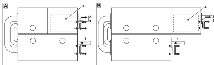
fig. 26 - Configurazioni contrapposte
