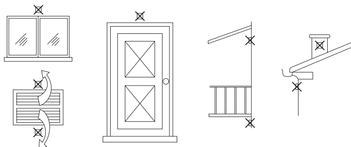
fig. 34 - Posizionamento sconsigliato sonda esterna
