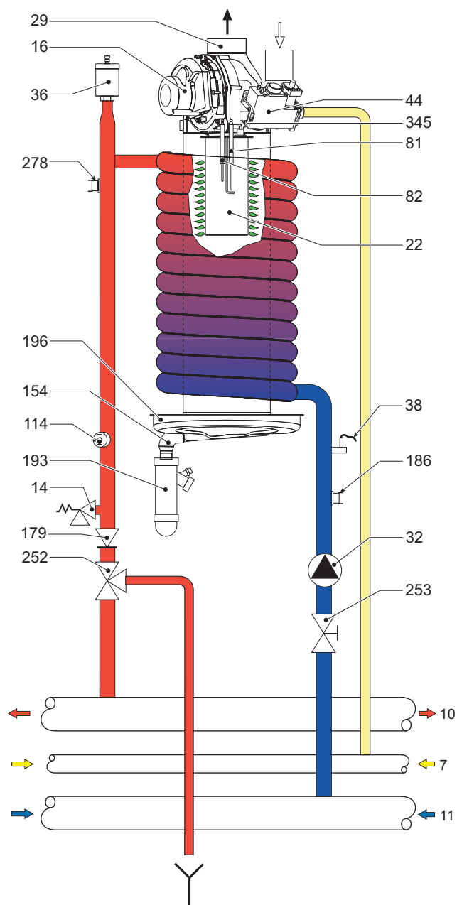
fig. 65 - Circuito idraulico modello FUTURIA POWER 80 - 125
