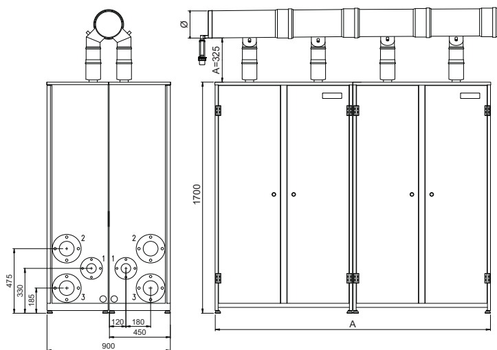
fig. 16 - Configurazione contrapposte
