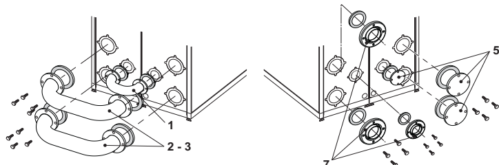
fig. 25 - Kit per il collegamento di moduli contrapposti
