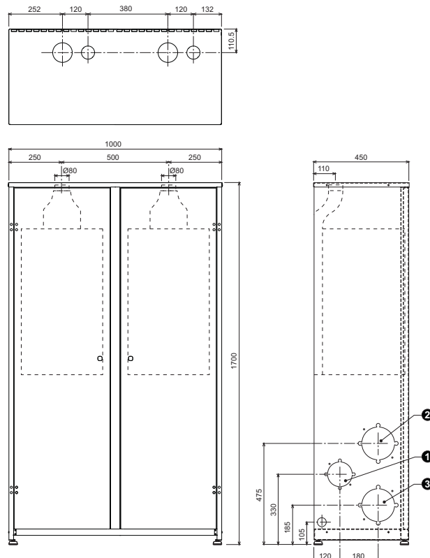
fig. 62 - Dimensione e attacchi modello FUTURIA POWER 160 - 250
