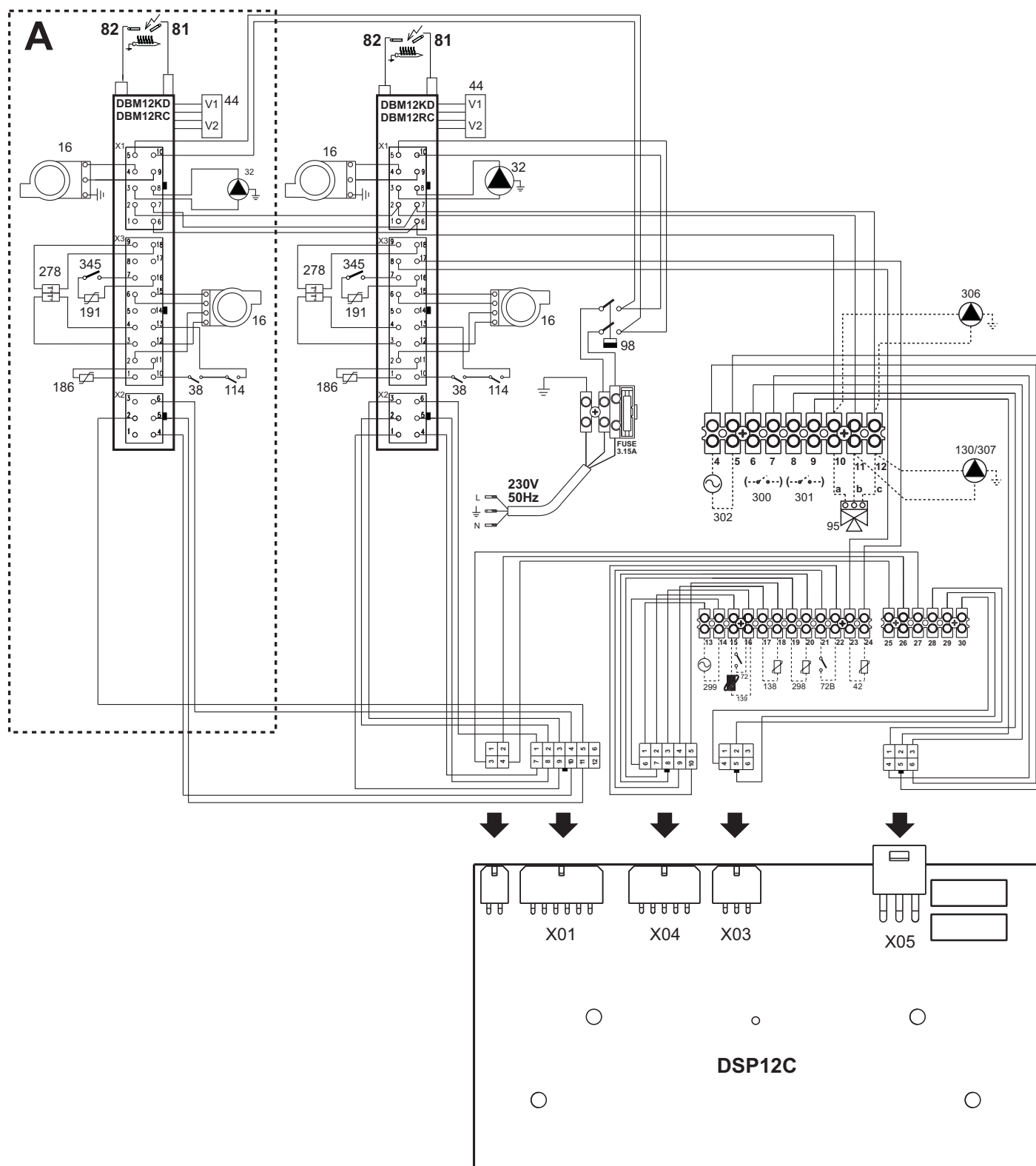
fig. 67 - Schema elettrico
