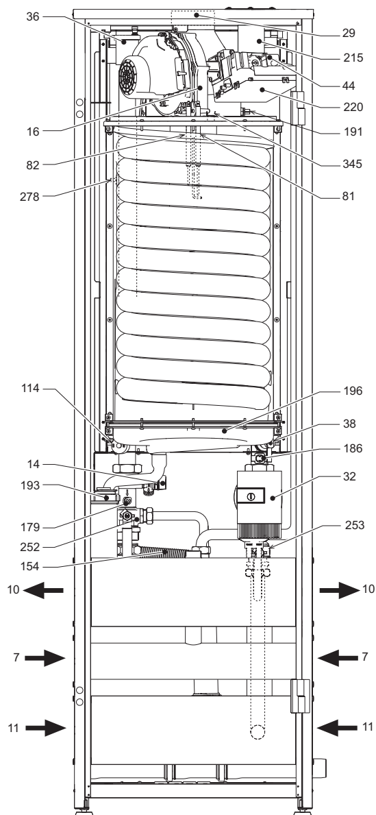
fig. 63 - Vista generale modello FUTURIA POWER 80 - 125
