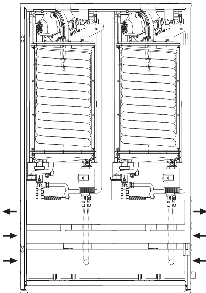
fig. 64 - Vista generale modello FUTURIA POWER 160 - 250
