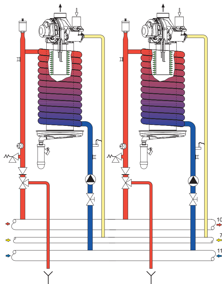
fig. 66 - Circuito idraulico modello FUTURIA POWER 160 - 250
