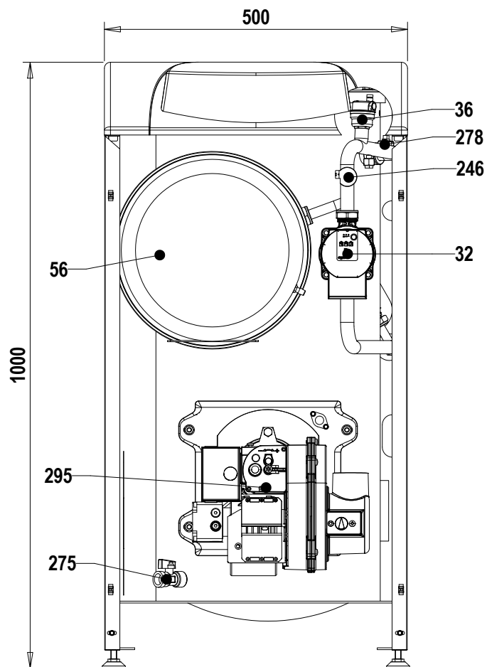
fig.35 - Vista frontal
