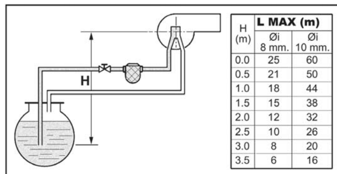
fig.20 - Alimentación por aspiración
