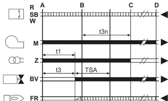
fig.31 - Ciclo dell'apparecchiatura
