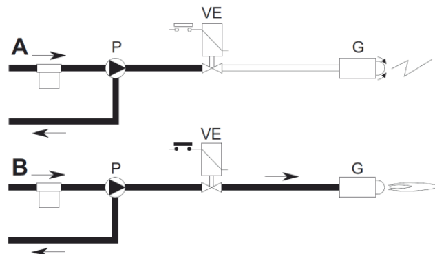
fig.30 - Avviamento
