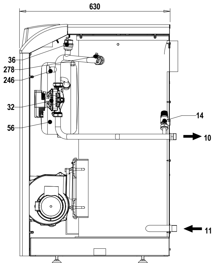
fig.36 - Vista laterale
