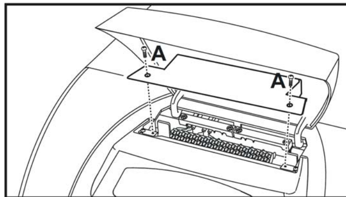
fig.23 - Acceso a la regleta de conexiones
