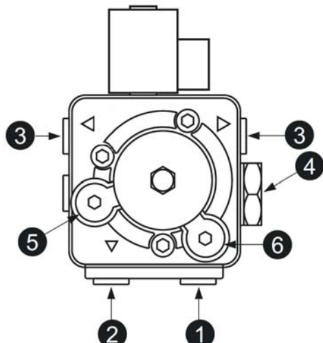
fig.25 - Bomba ITALPUMP
