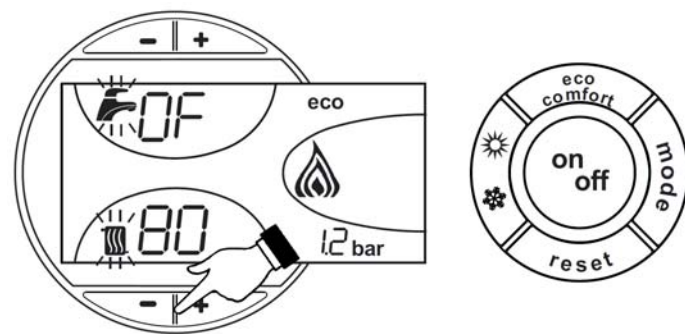
fig.24 - Modalità TEST
