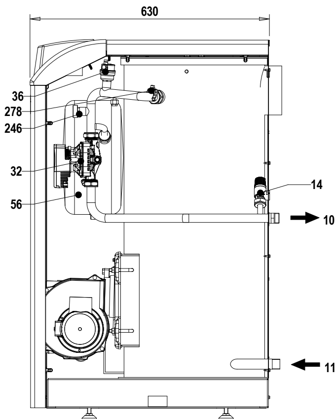
fig.36 - Vista lateral
