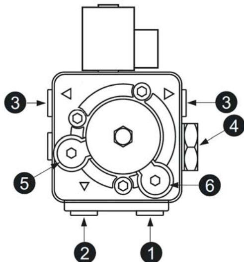
fig.25 - Pompa ITALPUMP
