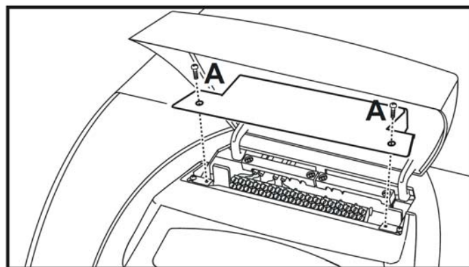
fig.23 – Accesso alla morsettiera
