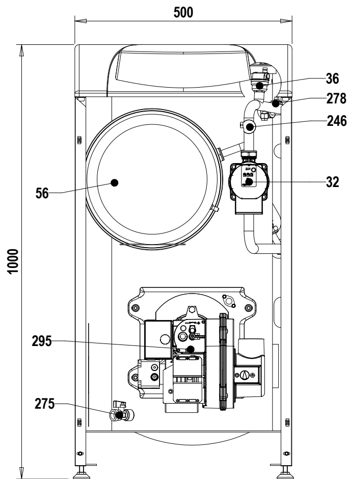
fig.35 - Vista frontale
