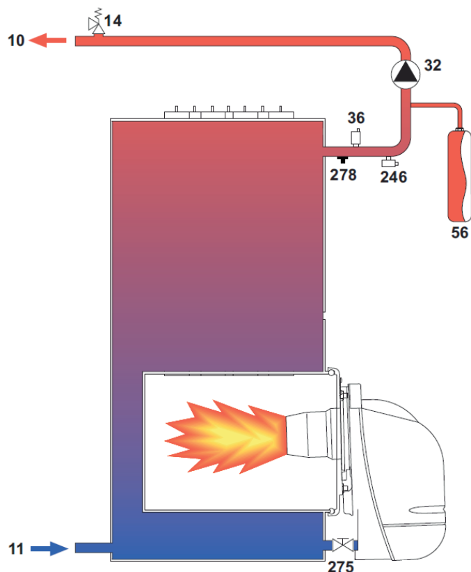
fig.38 - Circuito hidráulico
