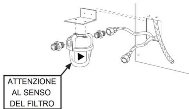
fig.19 - Installazione filtro combustibile
