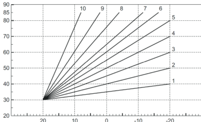
fig.14 – Curve di compensazione
