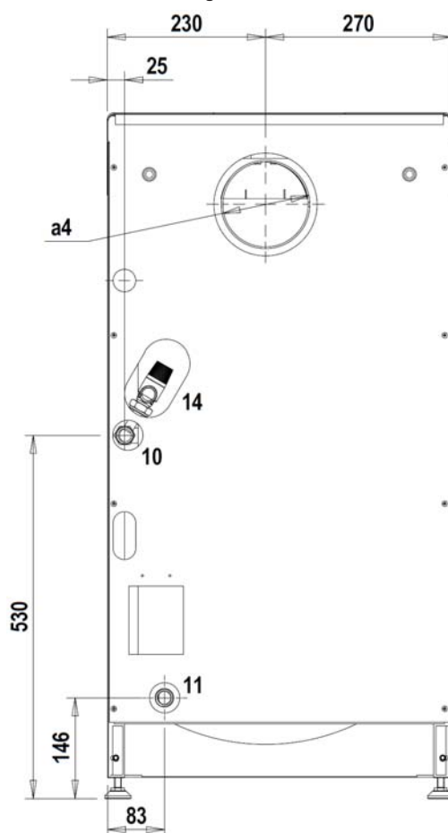
fig.36 - Vista lateral
