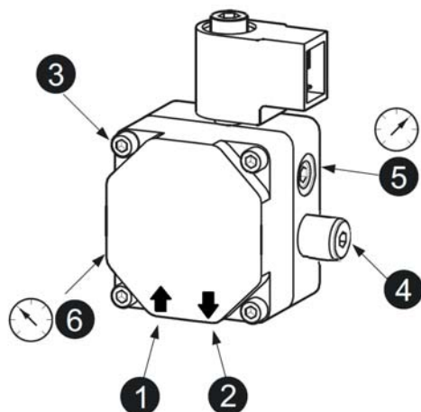
fig.26 - Pompa DANFOSS
