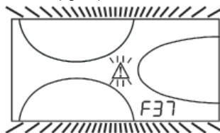
fig.16 - Anomalía por baja presión en la instalación
