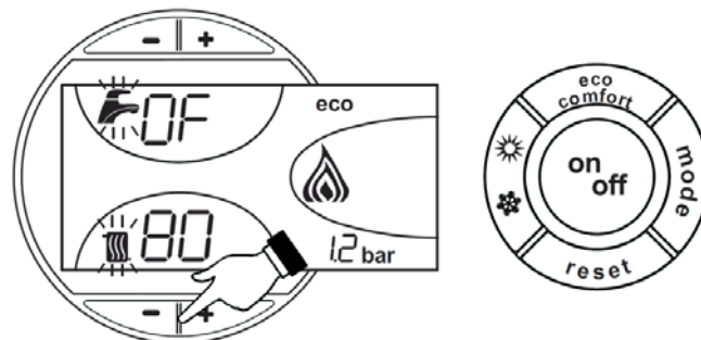
fig.24 - Modo TEST
