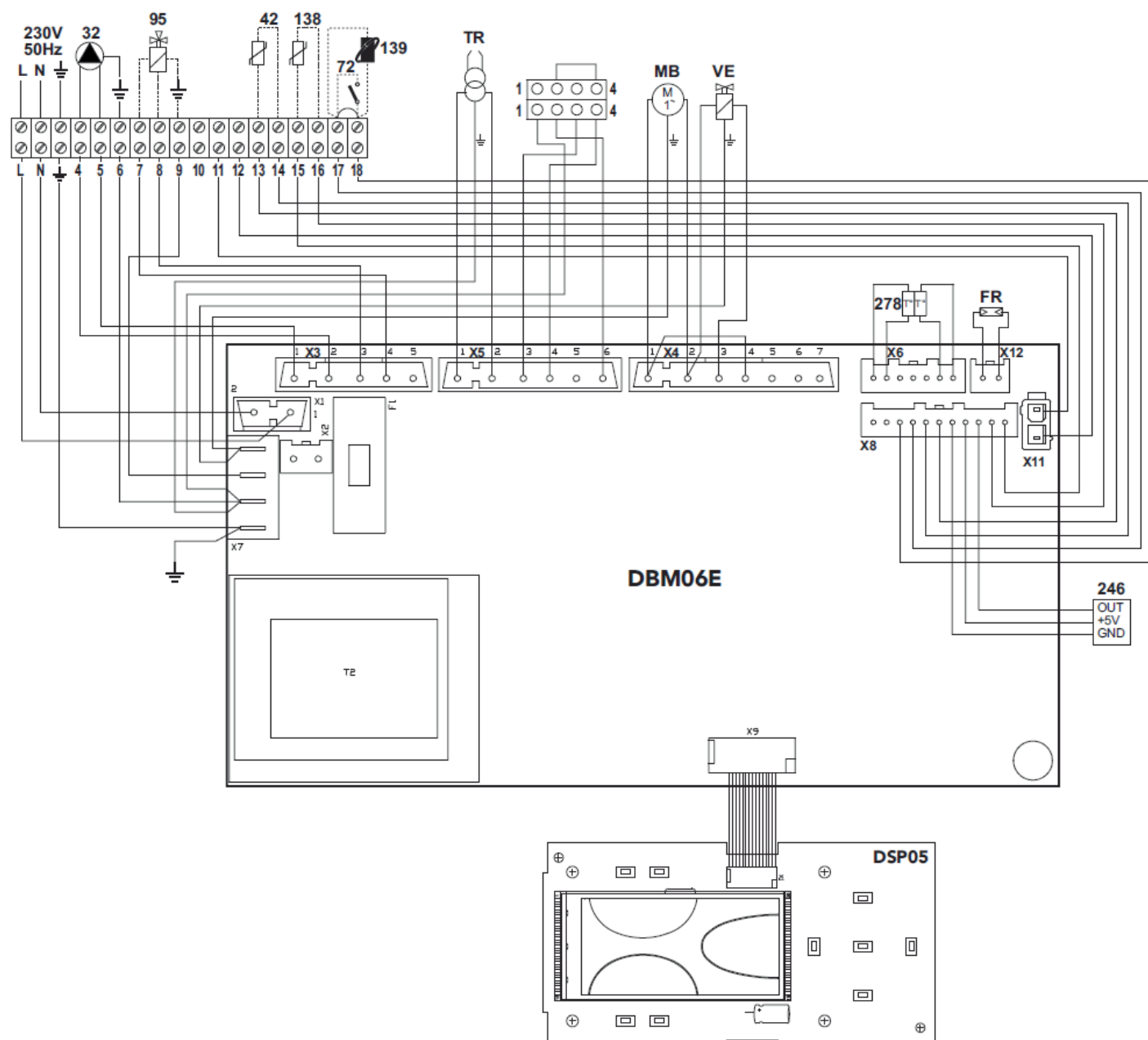
fig.41 - Esquema eléctrico
