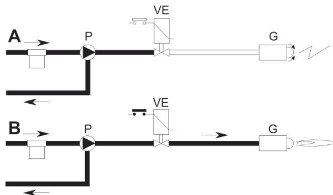
fig.30 - Encendido
