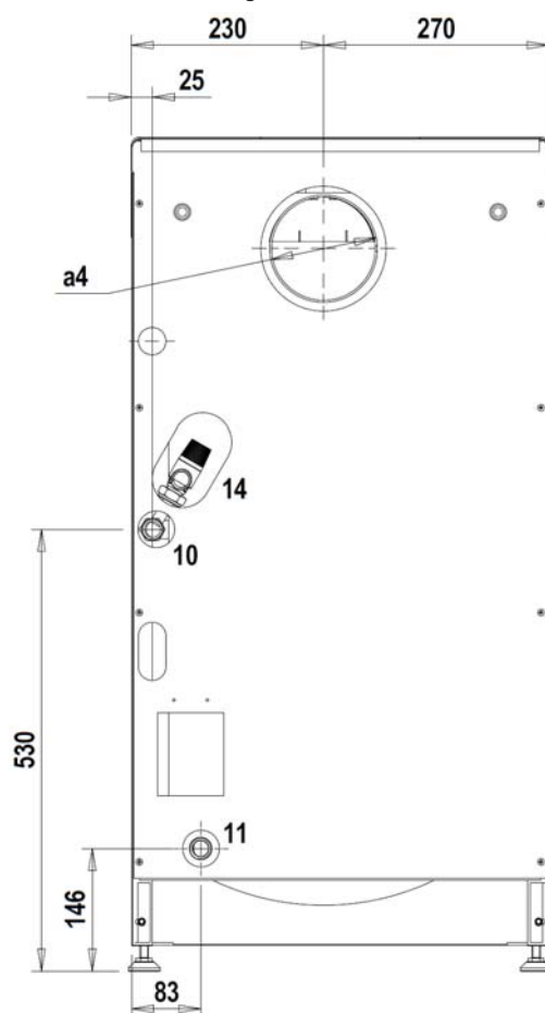
fig.36 - Vista laterale
