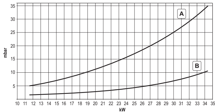
Диаграммы давление - мощность FL D C32
