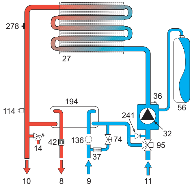
рис. 22- Контур отопления
