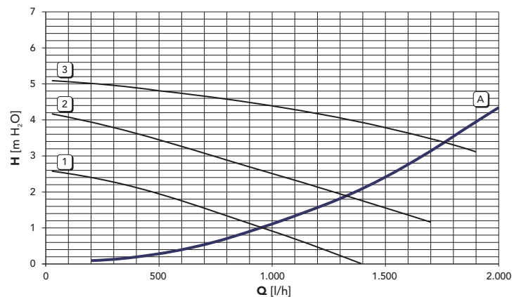
Потери нагрузки/напора циркуляционных насосов FL D C24
