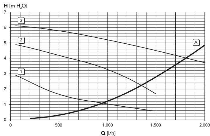
Потери нагрузки/напора циркуляционных насосов FL D C32
