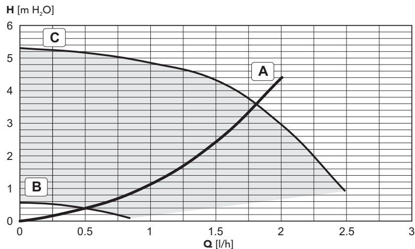
рис. 32 - Потери нагрузки/напор циркуляционного насоса SILVER 24C
