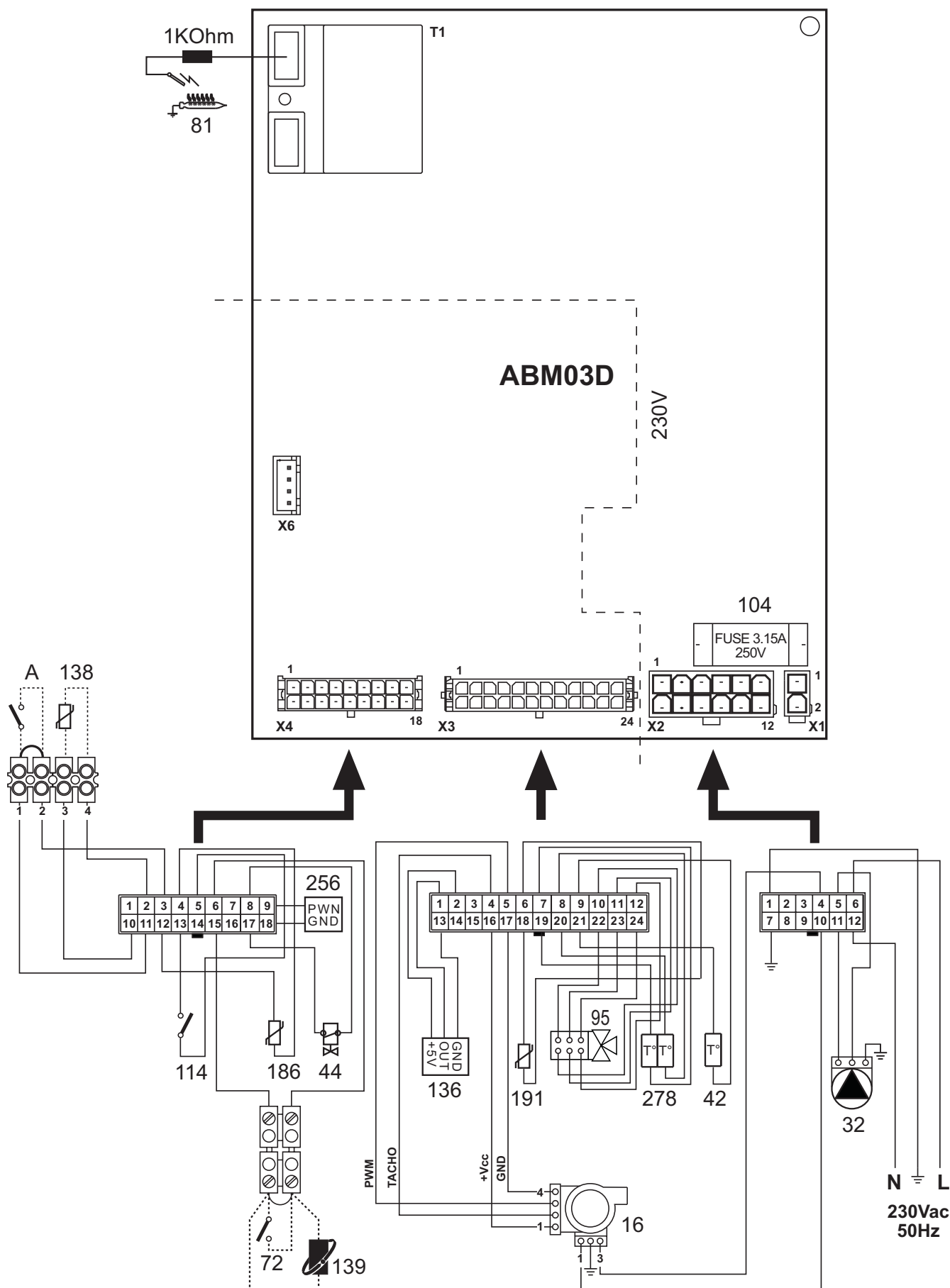
fig. 34 - Esquema eléctrico
