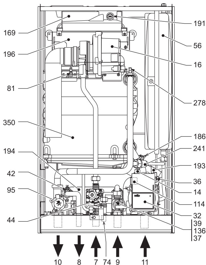
рис. 30 - Общий вид
