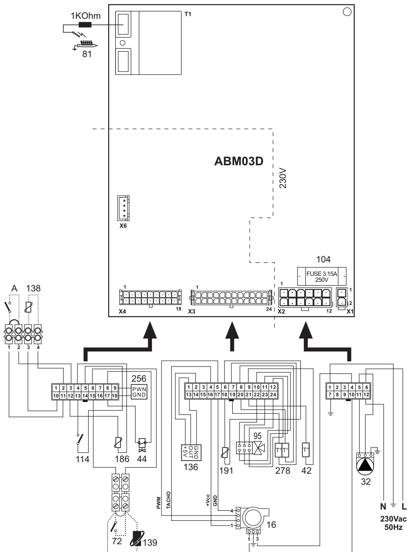
fig. 34 - Wiring diagram
