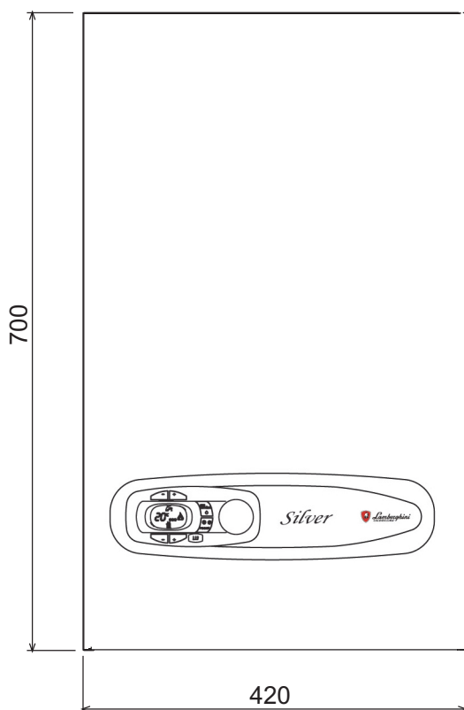
fig. 26 - Vista frontale
