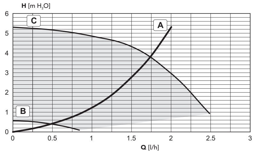
fig. 33 - Pertes de charge/pression circulateur SILVER 34C
