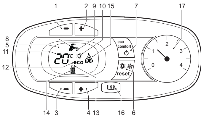
рис. 1 - Панель управления
