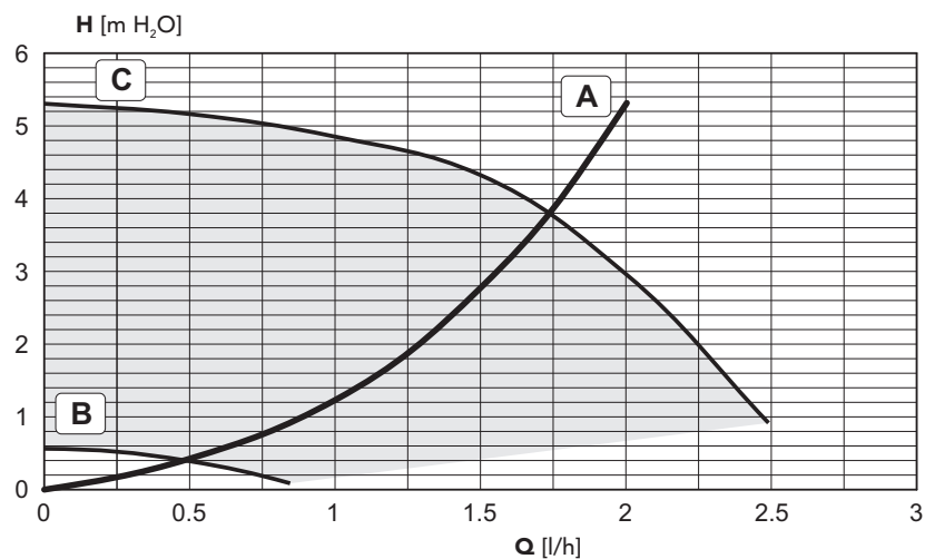
fig. 33 - Pérdidas de carga / altura de impulsión circulador SILVER 34C
