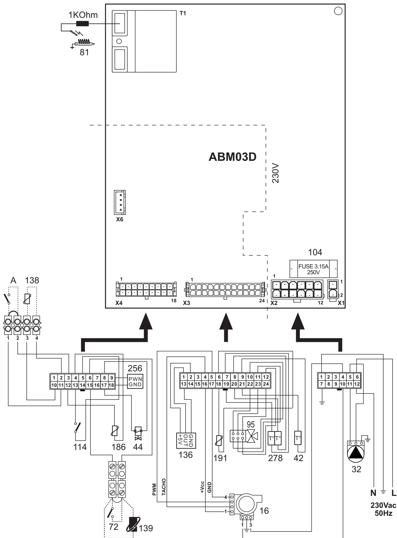
fig. 34 - Schéma électrique
