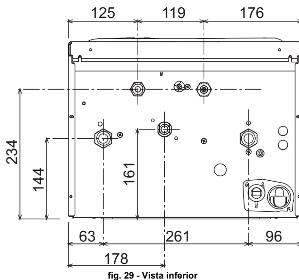
fig. 29 - Vista inferior
