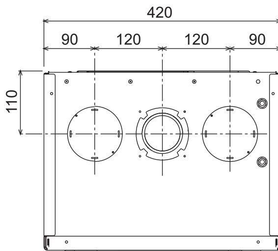
fig. 28 - Vista dall'alto
