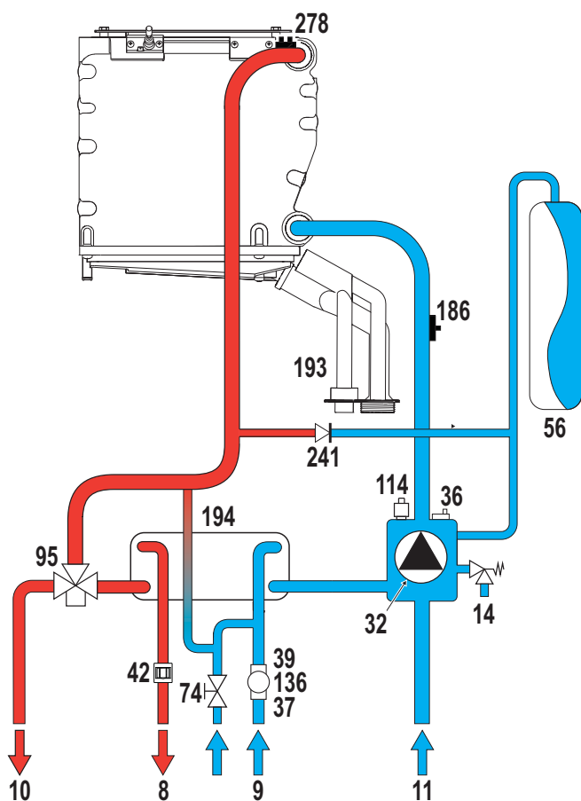
fig. 31 - Circuito idraulico
