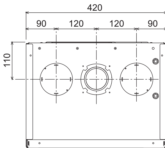
рис. 28 - Вид сверху
