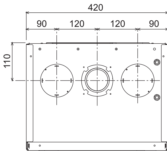
fig. 28 - Vista superior
