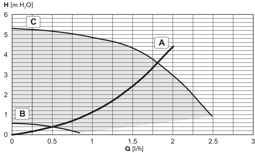
fig. 32 - Pertes de charge/pression circulateur SILVER 24C
