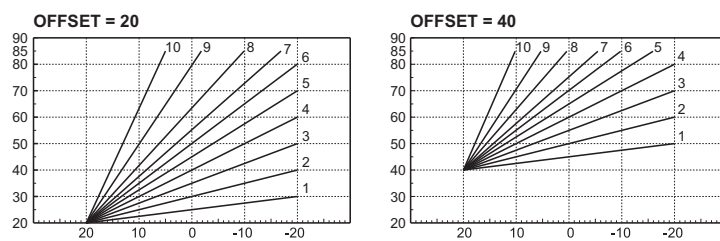
fig. 12 - Ejemplo de desplazamiento paralelo de las curvas de compensación
