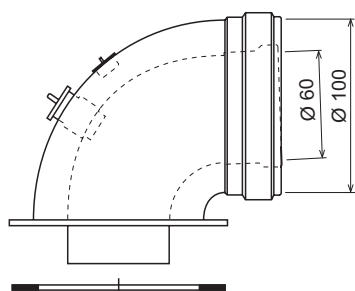
fig. 16 - Accessori di partenza per condotti coassiali
