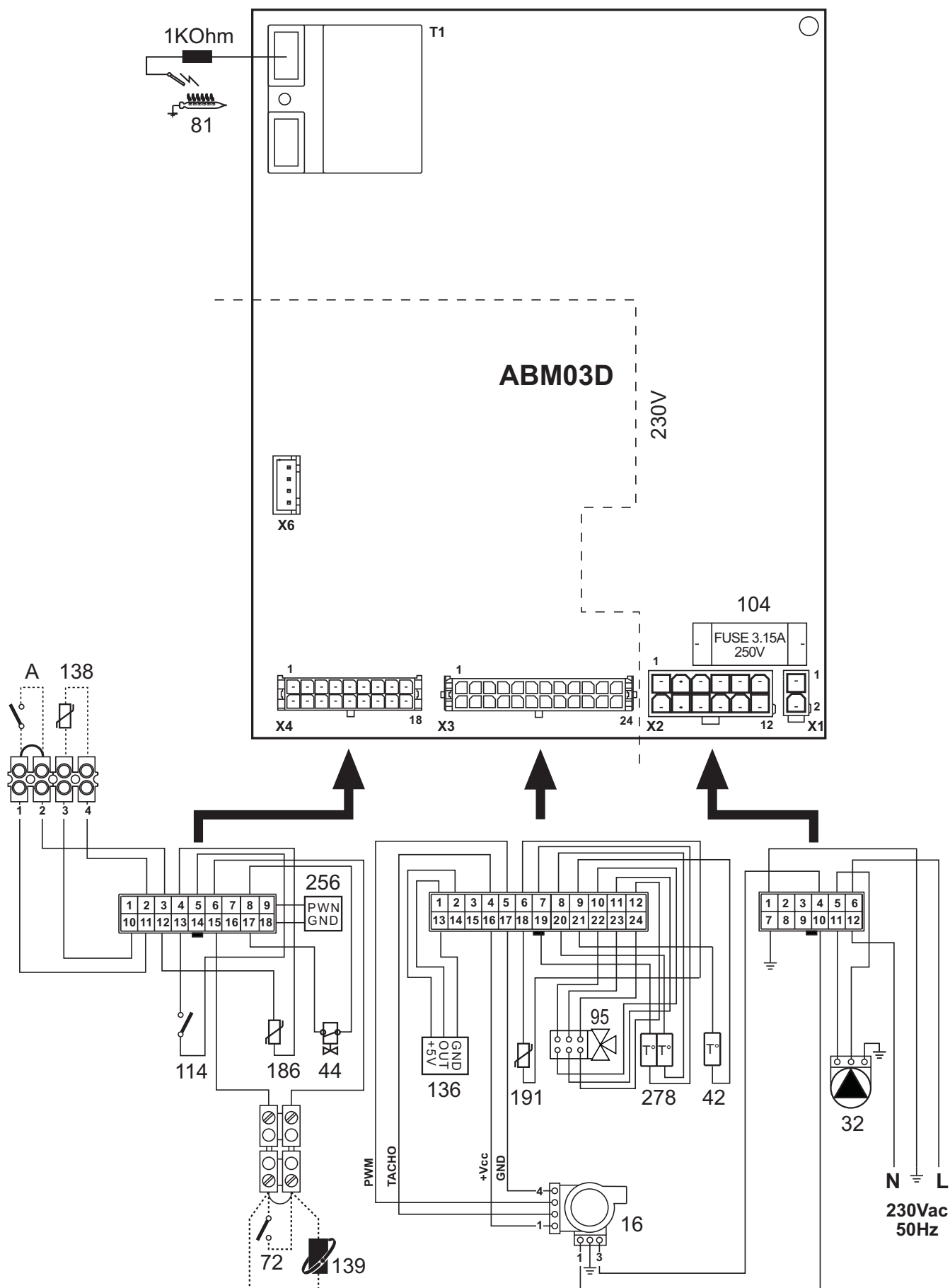
fig. 34 - Schema elettrico
