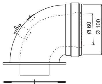
рис. 16 - Элементы для коаксиальных воздухопроводов
