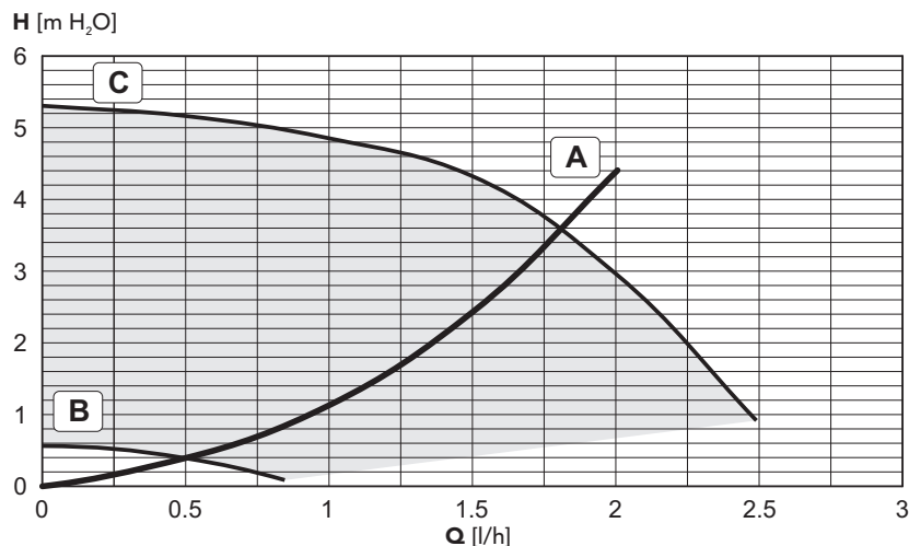
fig. 32 - Pérdidas de carga/altura de impulsión circulador SILVER 24C
