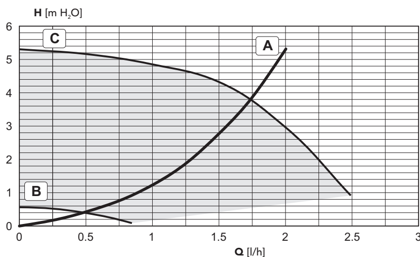
рис. 33 - Потери нагрузки/напор циркуляционного насоса SILVER 34C
