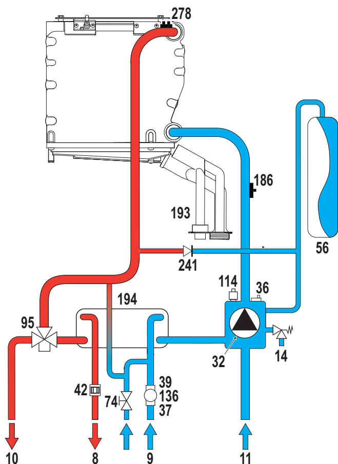
fig. 31 - Circuito hidráulico
