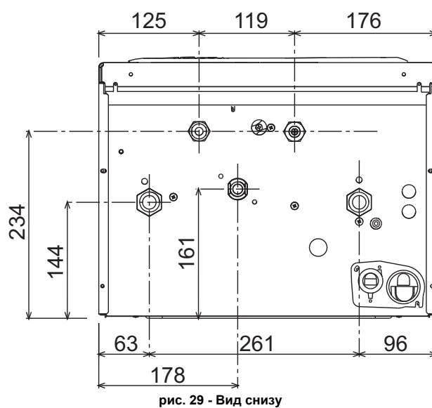
рис. 29 - Вид снизу
