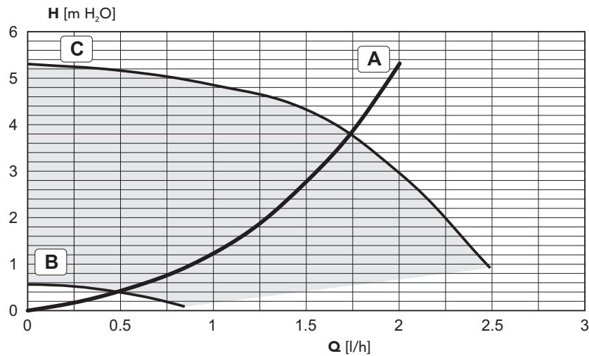
fig. 33 - Perdite di carico / prevalenza circolatore SILVER 34C
