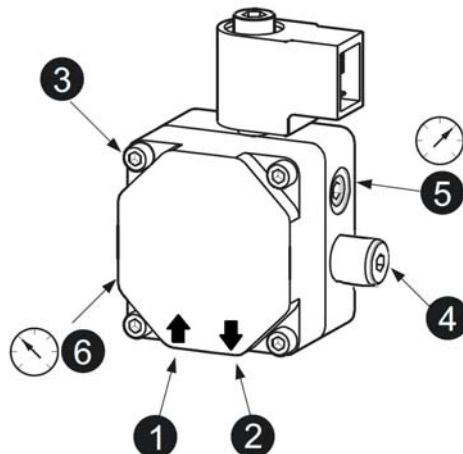
fig.27 - Pompa DANFOSS
