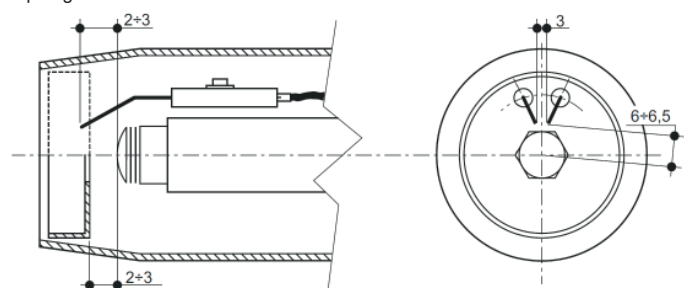
fig.30 - Posizione elettrodi - deflettore
