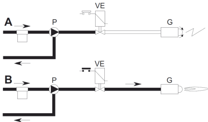
fig.31 - Avviamento
