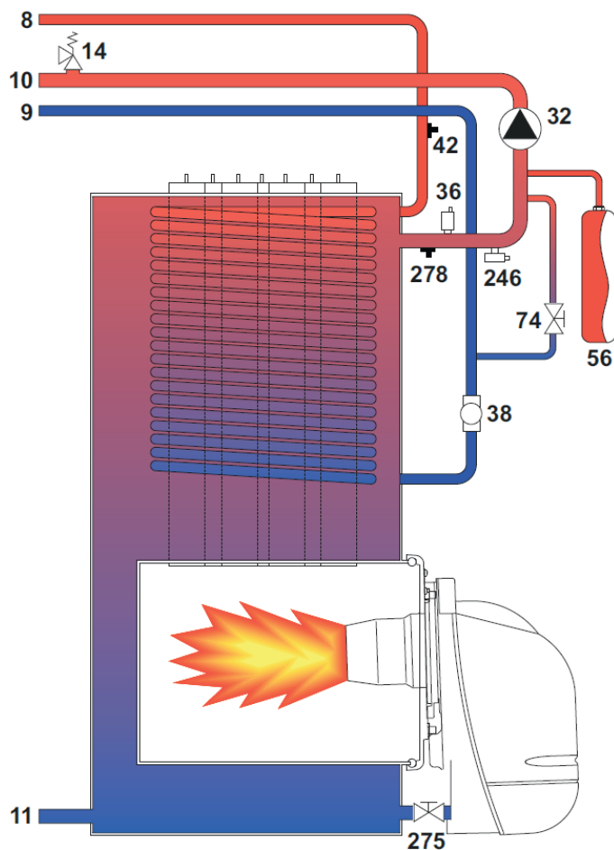
fig.40 - Circuito idraulico
