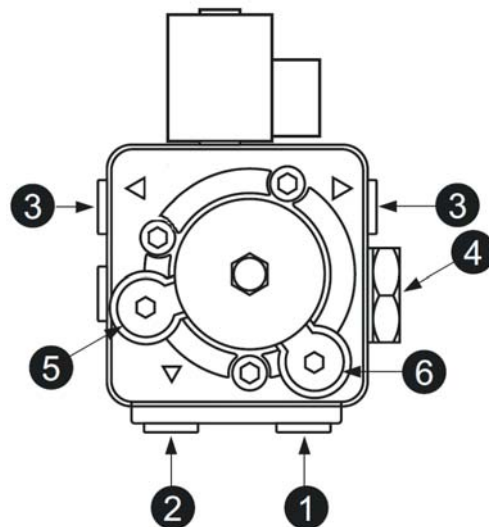
fig.26 - Pompa ITALPUMP
