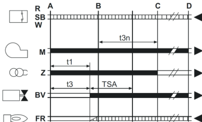
fig.32 - Ciclo dell'apparecchiatura
