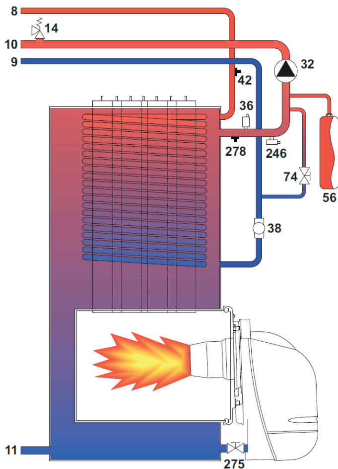
fig.40 - Circuito hidráulico
