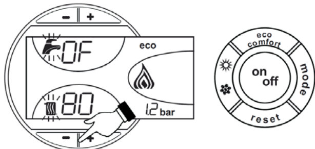
fig.25 - Modalità TEST
