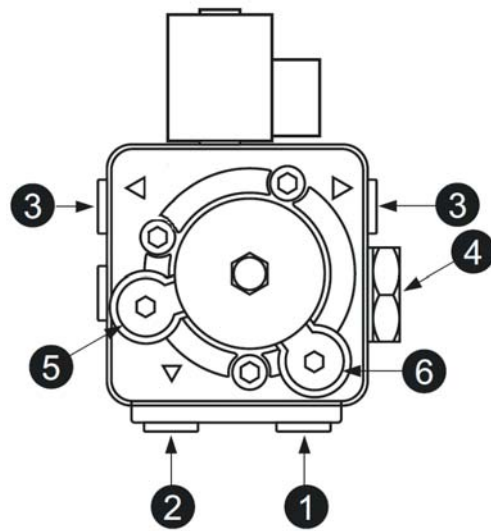
fig.26 - Bomba ITALPUMP
