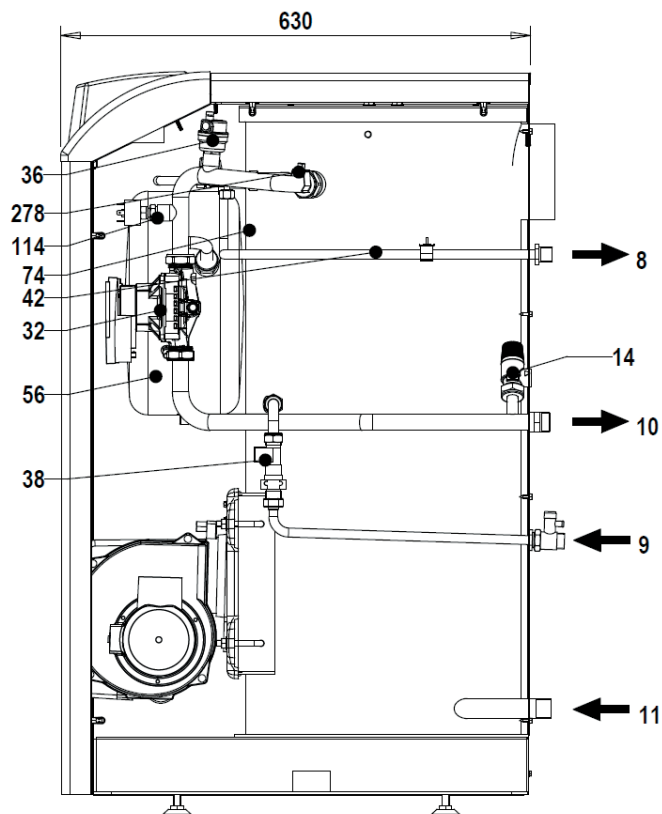
fig.38 - Vista laterale
