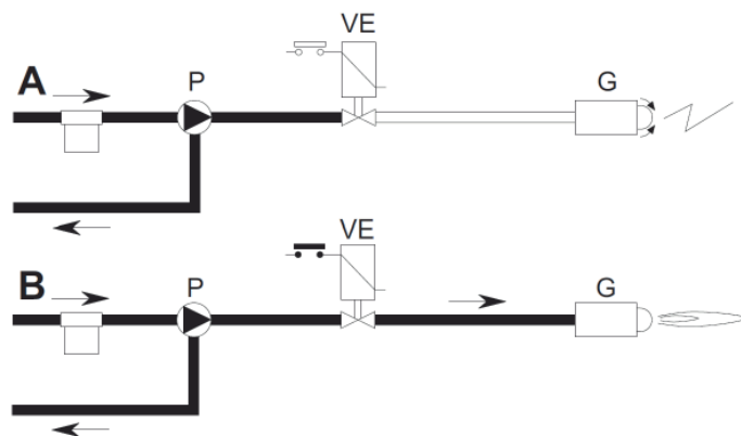
fig.31 - Encendido
