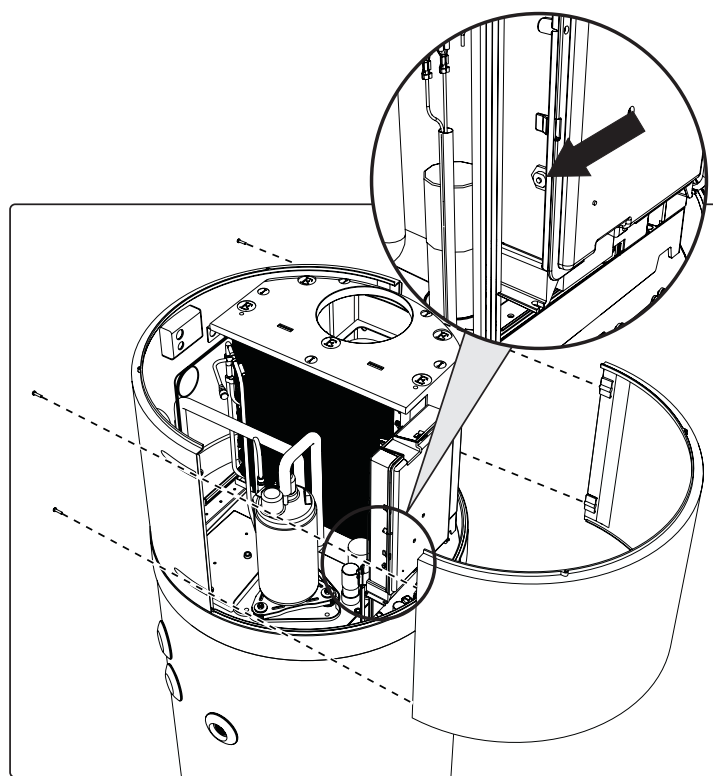
fig. 42 - Rimozione pannello frontale
