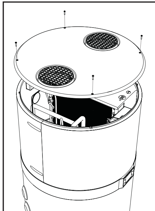
fig. 41 - Rimozione copertura superiore
