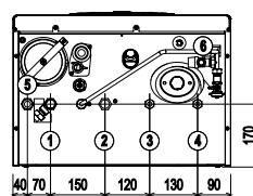
Vista inferiore
