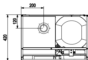
Vista superiore
