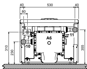
VISTA DAL BASSO mod. TORO W 99 E 120
