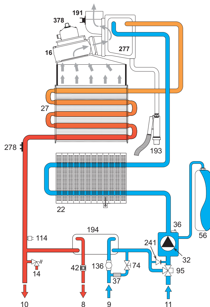
fig. 27- Circuitul de încălzire
