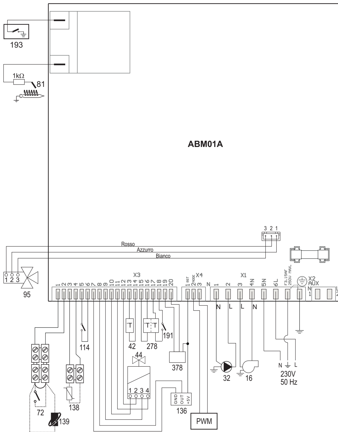
fig. 28 - Schema elettrico
