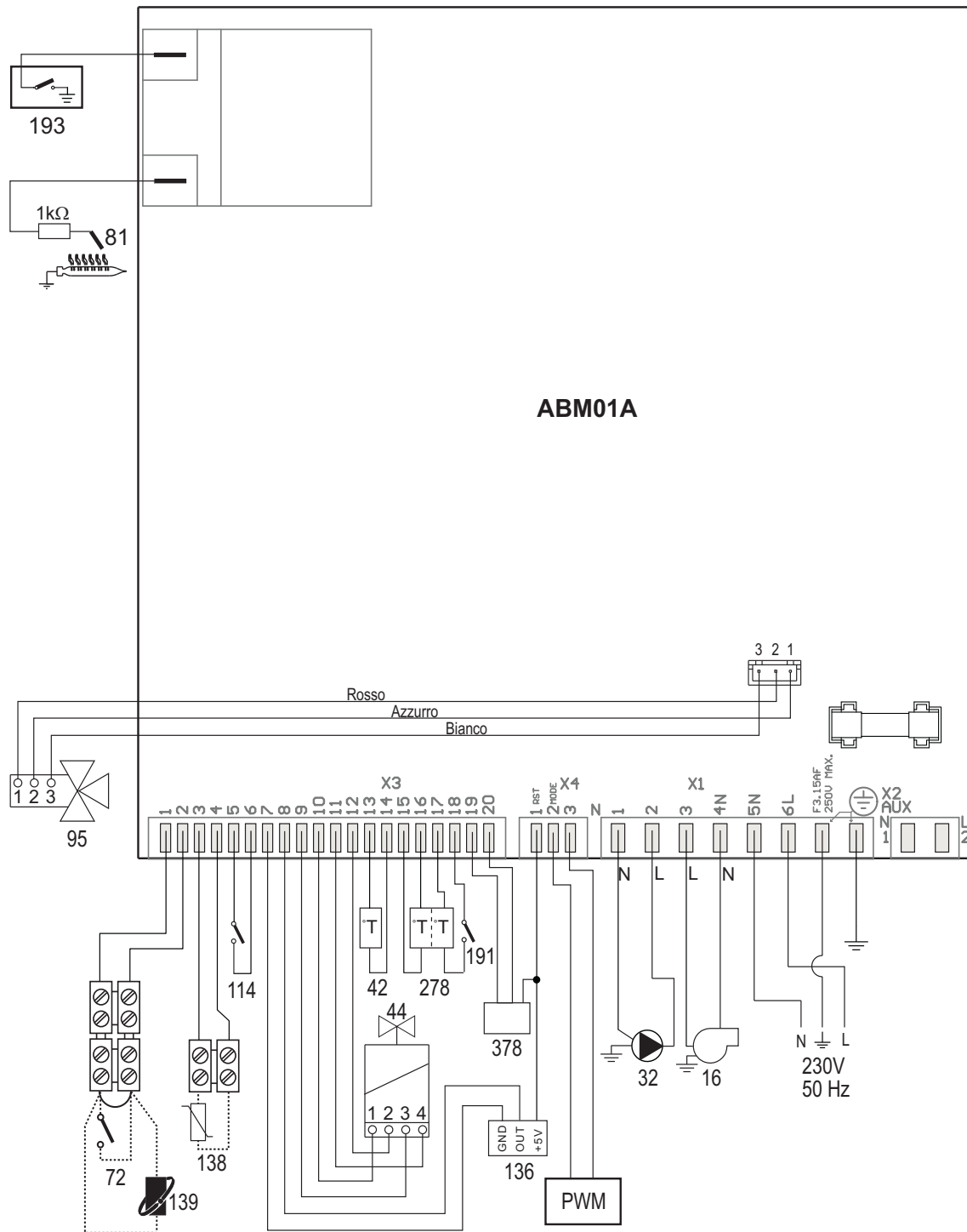
fig. 28- Esquema eléctrico
