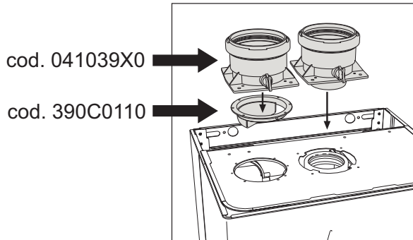
εικ. 15 - Εξάρτημα σύνδεσης για ξεχωριστούς αγωγούς
