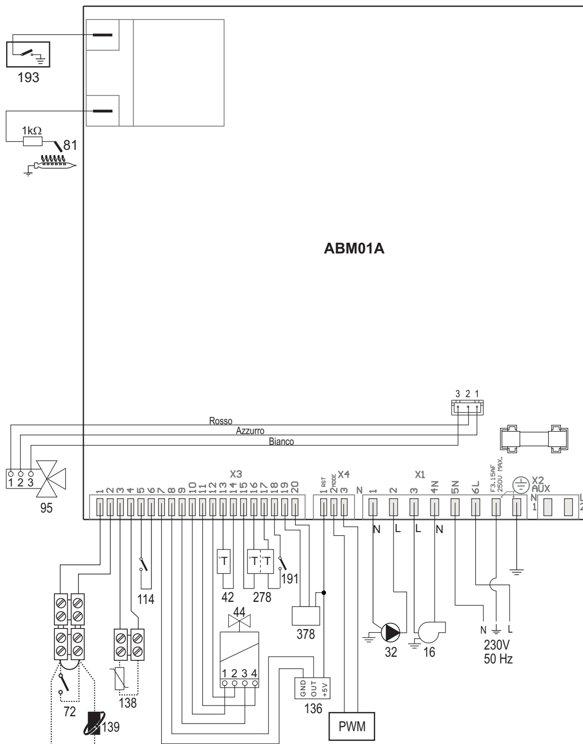
fig. 28- Schemă electrică
