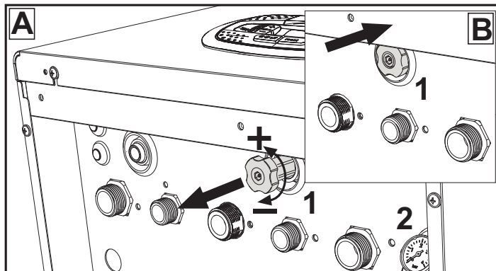
wygląd 8 - Pokrętło napełniania
