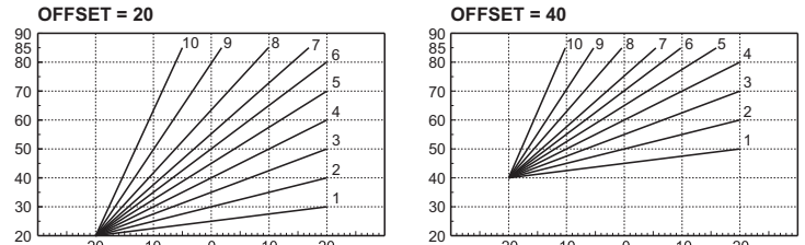
fig. 7 - Ejemplo de desplazamiento paralelo de las curvas de compensación
