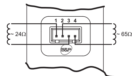
fig. 18 - Conexiune valvă gaz
