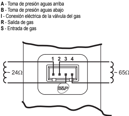
fig. 18 - Conexión de la válvula de gas
