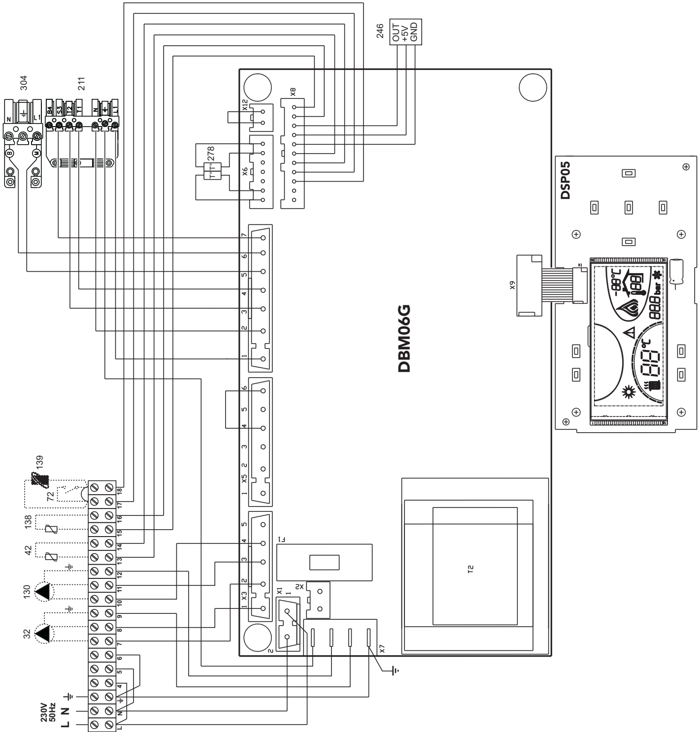
fig. 23 - Wiring diagram
