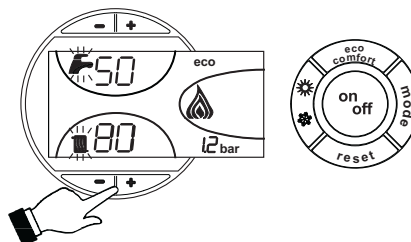
fig. 18 - Mode TEST
