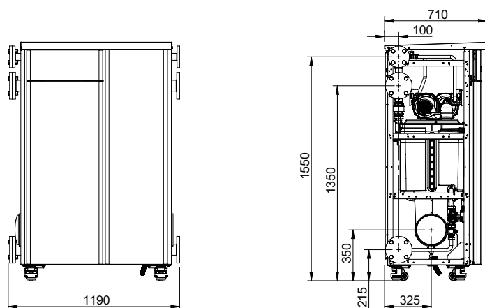
mod. 150 - 225 - 300
