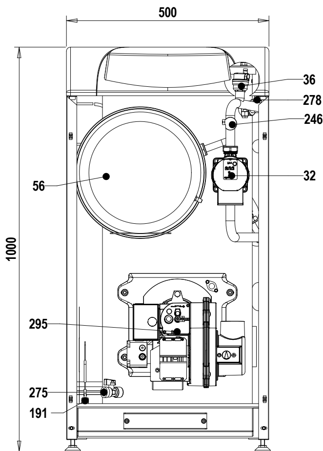
fig.38 - Vista frontale
