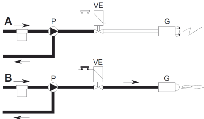
fig.31 - Avviamento
