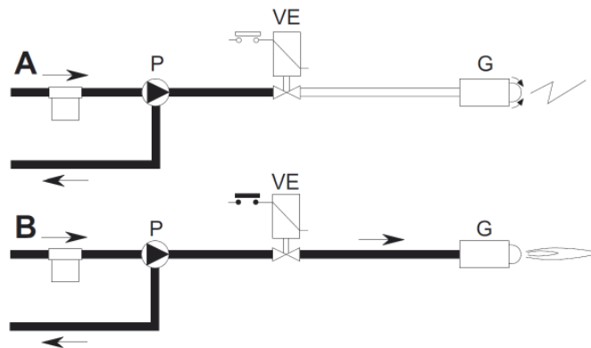
fig.31 - Encendido
