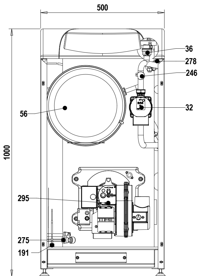
fig.38 - Vista frontal
