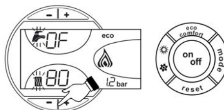
fig.25 – Modo TEST
