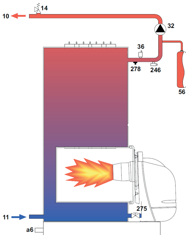
fig.40 – Circuito hidráulico
