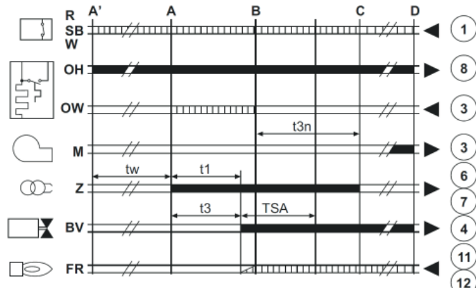
fig.32 - Ciclo dell'apparecchiatura
