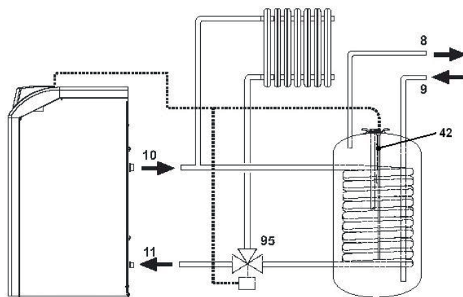
fig.18 - Schema collegamento ad un bollitore esterno
