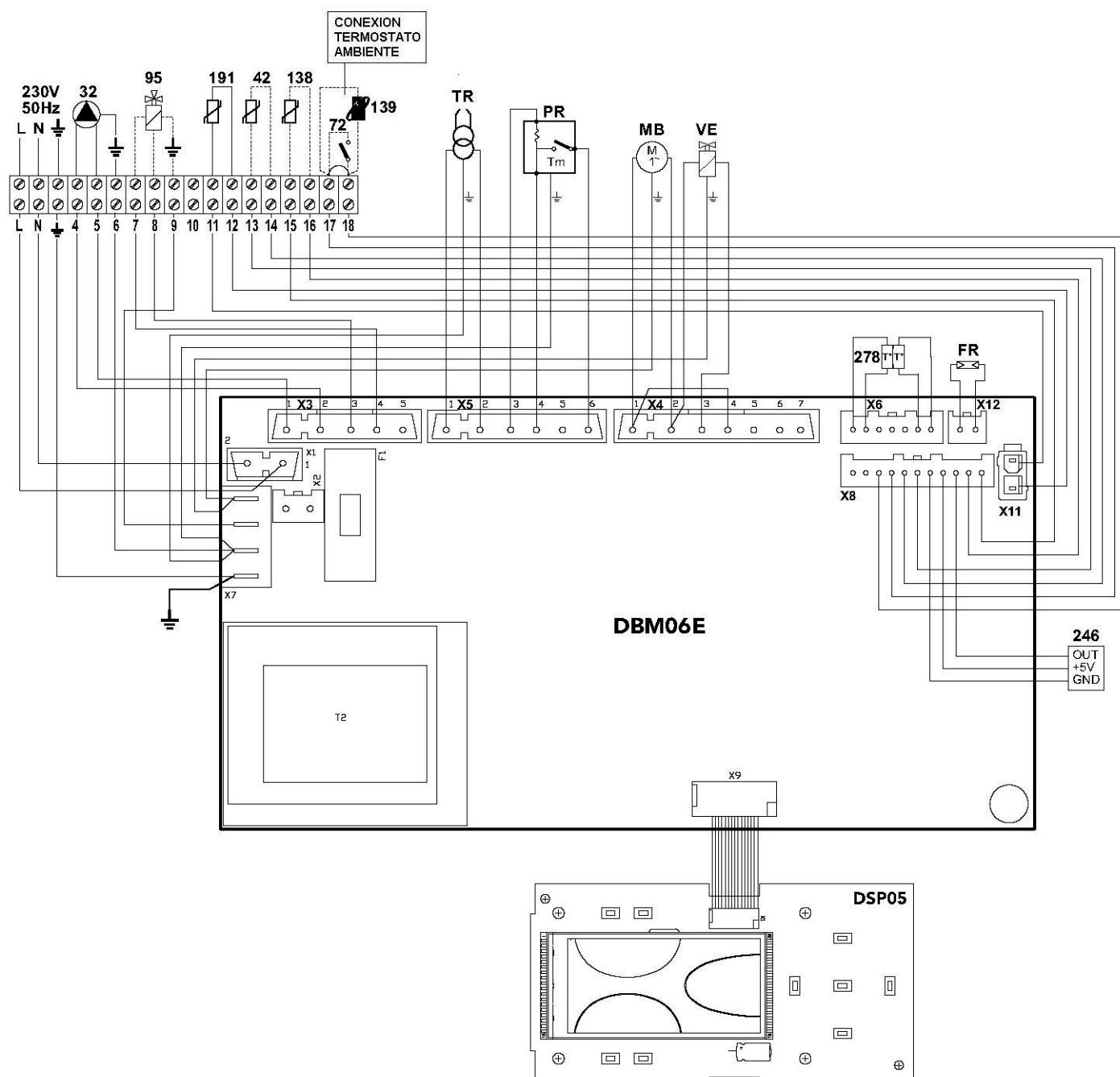
fig.43 – Esquema eléctrico
