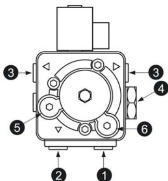
fig.26 - Pompa ITALPUMP
