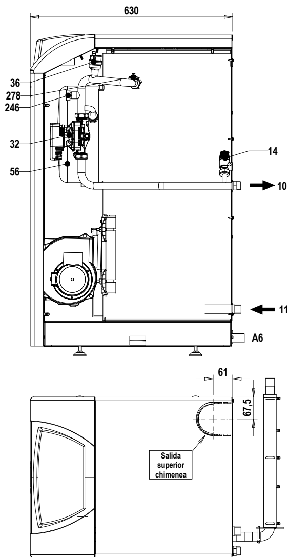
fig.37 - Vista lateral y superior
