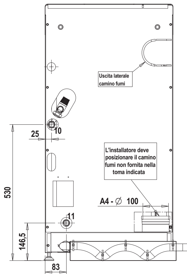
fig.39 - Vista posteriore
