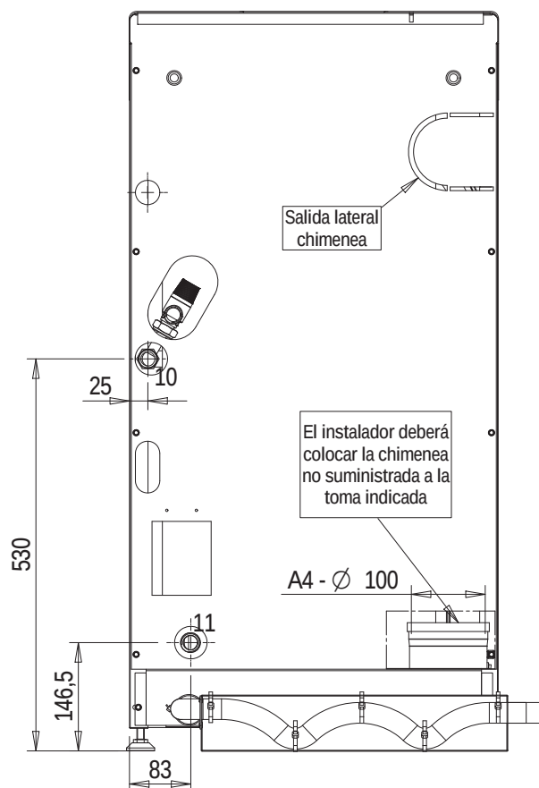
fig.39 - Vista posterior
