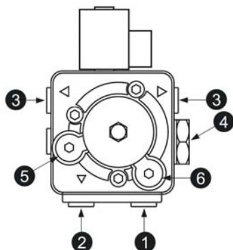
fig.26 - Bomba ITALPUMP
