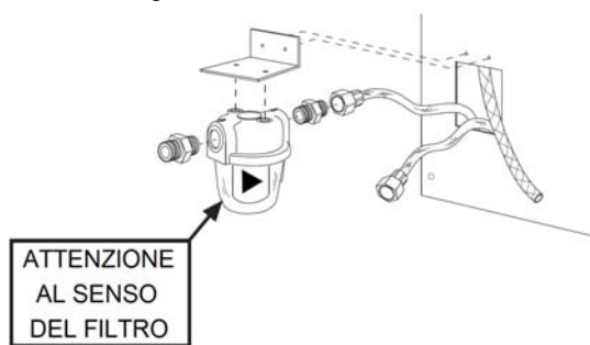
fig.19 - Installazione filtro combustibile
