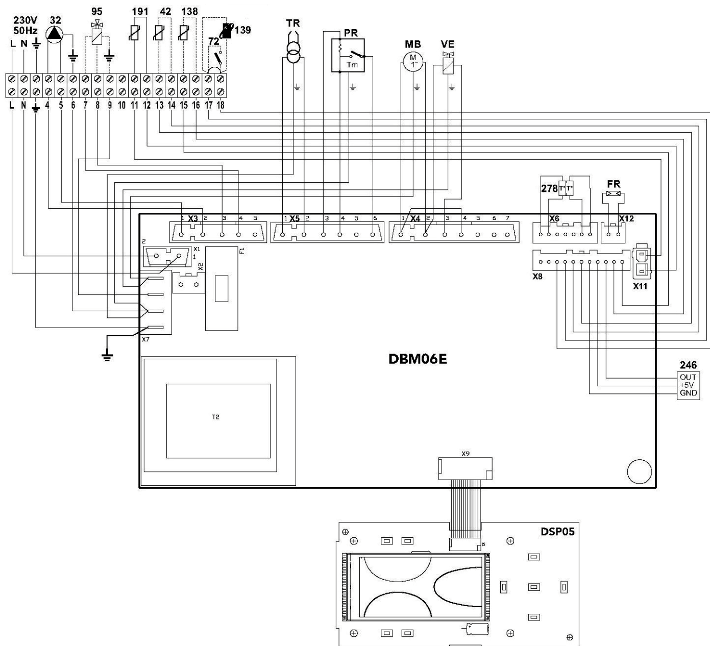
fig.43 – Esquema eléctrico
