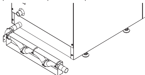
fig.24 – Scarico condensa
