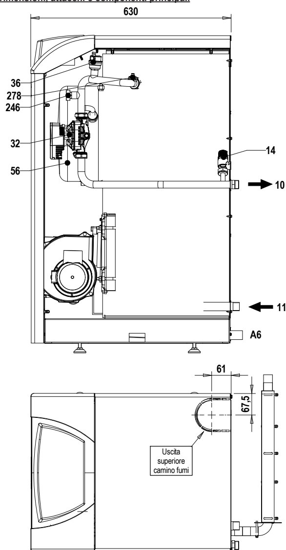
fig.37 - Vista laterale e superiore
