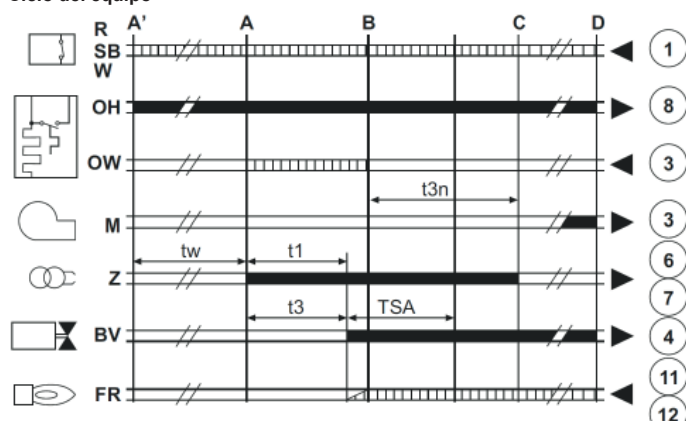
fig.32 - Ciclo del equipo
