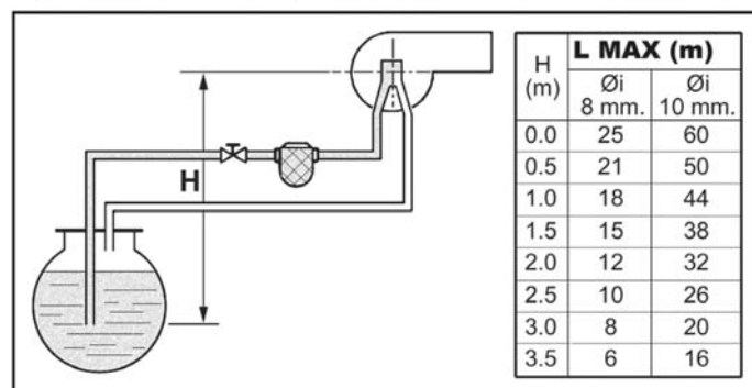
fig.20 - Alimentazione per gravità
