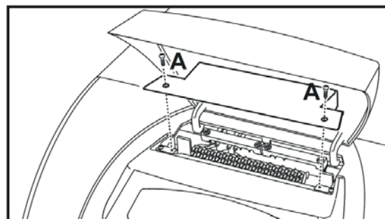
fig.23 – Accesso alla morsettiere
