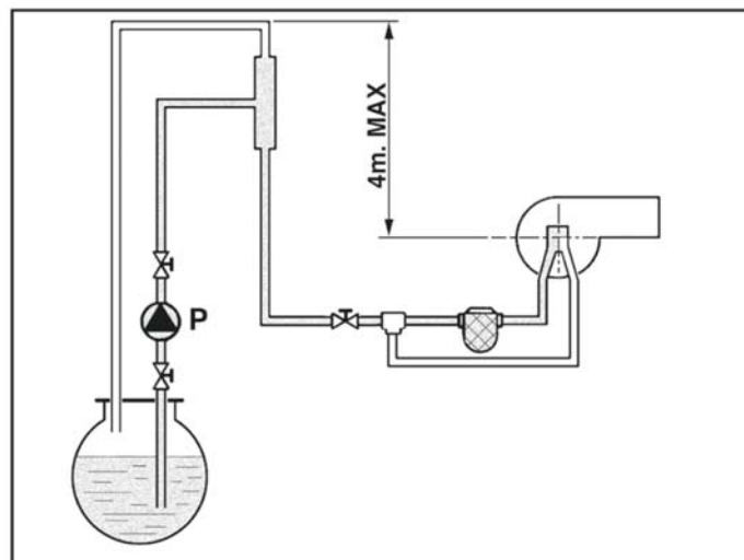
fig.22 – Alimentazione ad anello
