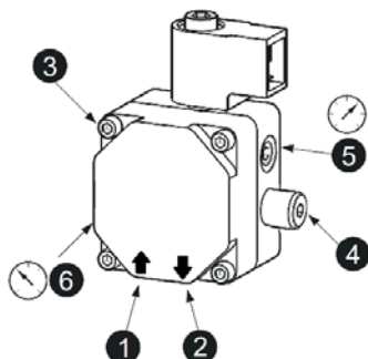
fig.27 - Pompa DANFOSS
