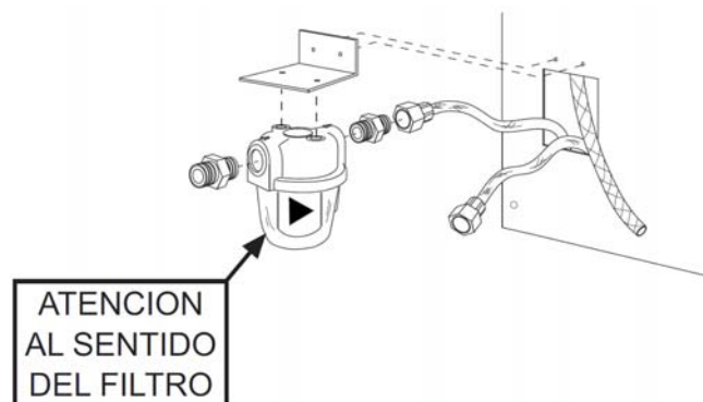
fig.19 - Instalación del filtro del combustible
