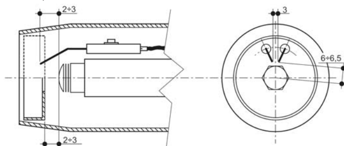
fig.30 - Posición de los electrodos y del deflector
