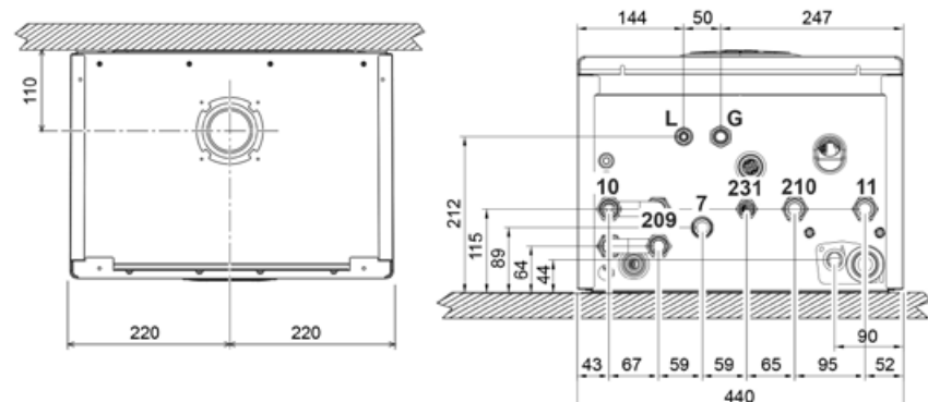
CONNESSIONI UNITÀ INTERNA IDOLA S HYBRID C
