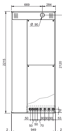
VISTA FRONTALE
