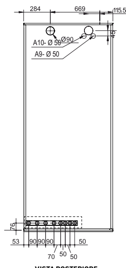
VISTA POSTERIORE
