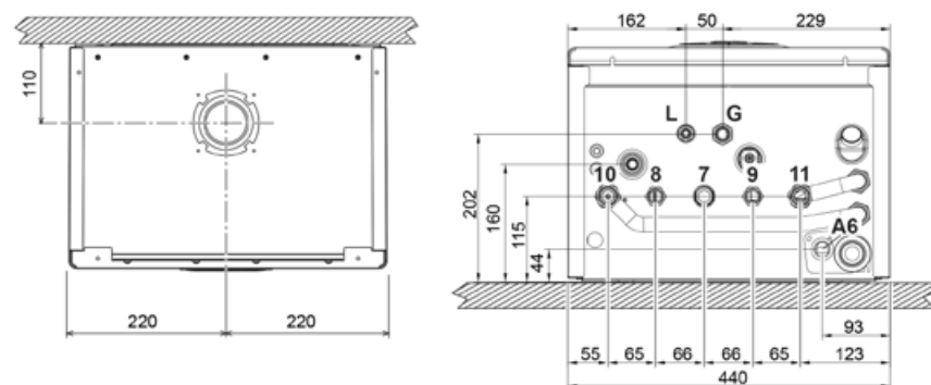
CONNESSIONI UNITÀ INTERNA IDOLA S HYBRID C
