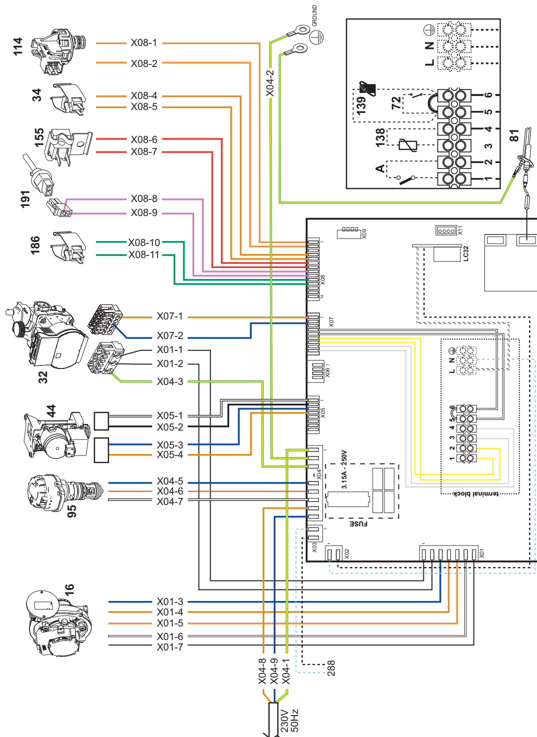
fig. 42 - Schema elettrico
