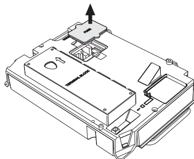
fig. 33 - Alloggiamento fusibile
