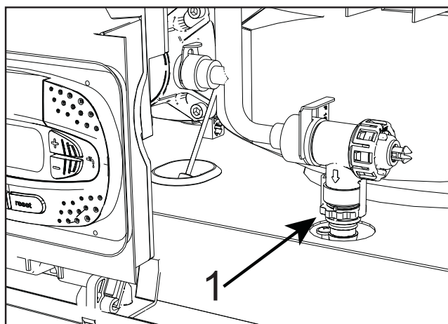
fig. 17 - Valvola di sicurezza con rubinetto di scarico
