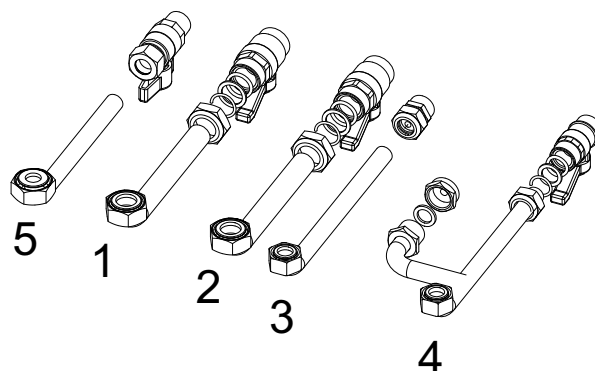
fig. 18 - Kit idraulico
