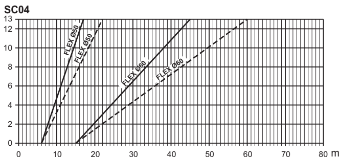
fig. 23- Grafic pentru alegerea parametrului pentru horn
