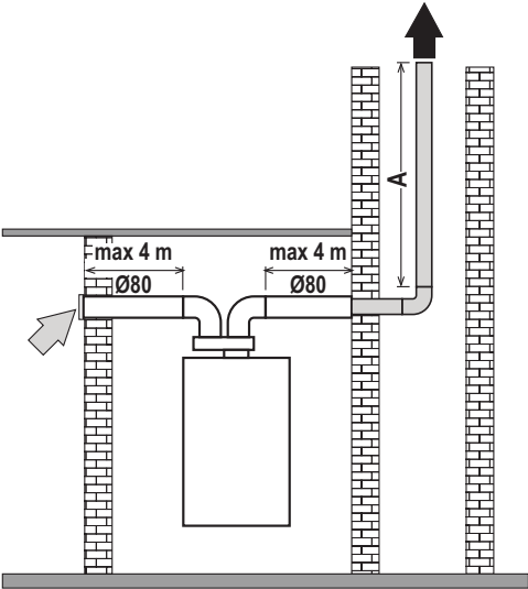
fig. 22- Esquema solo para entubamiento con flexible
