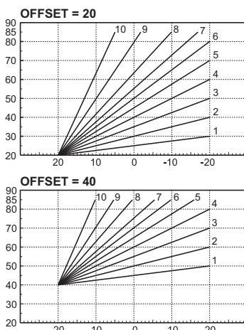
fig. 39 - Esempio di spostamento parallelo delle curve di compensazione
