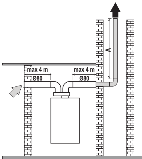
fig. 22 - Schema per solo intubamento con tubo flessibile
