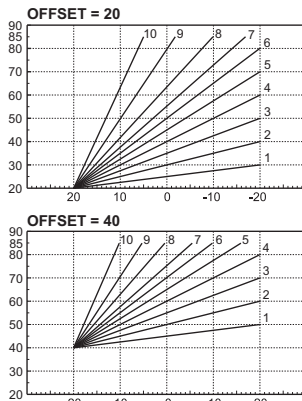
fig. 38- Ejemplo de desplazamiento paralelo de las curvas de compensación
