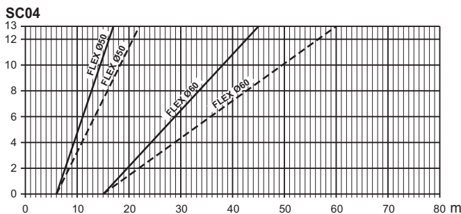
fig. 23- Chart for flue parameter choice
