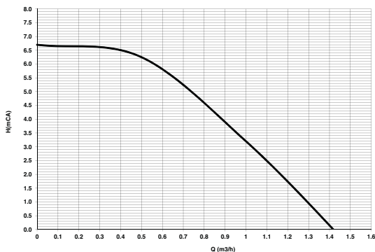
fig. 56- Carga hidrostática residual disponible en la instalación
