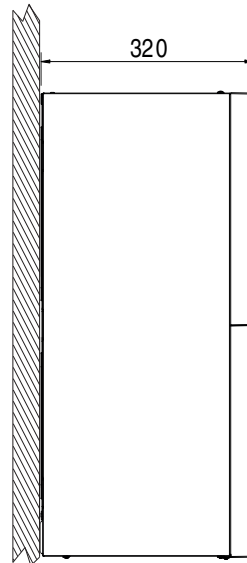
fig. 48- Vista lateral
