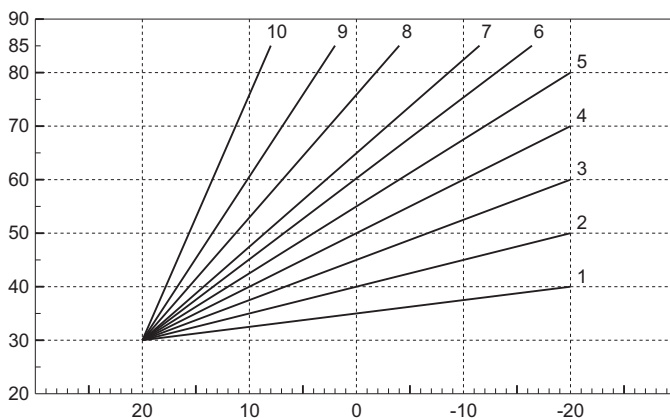
fig. 38 - Curve di compensazione
