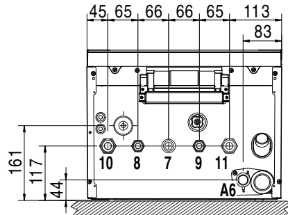
fig. 50- Vista inferior
