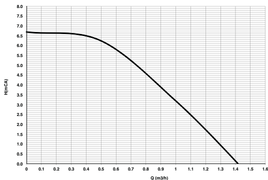
fig. 56- Înălțime de pompare reziduală disponibilă în instalație
