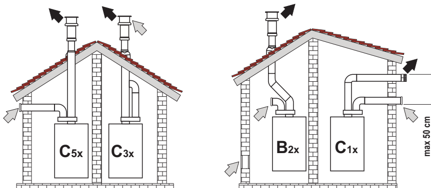
fig. 18 - Esempi di collegamento con tubi separati
