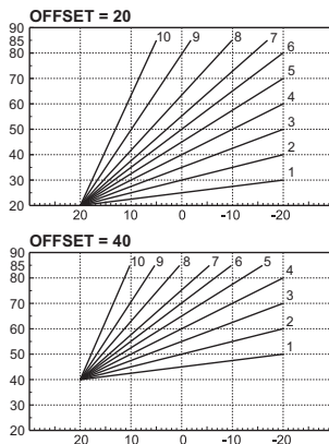
fig. 38- Exemplu de deplasare paralelă a curbelor de compensare
