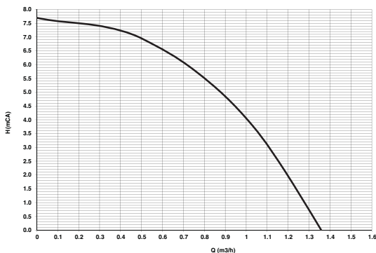
fig. 57- Înălțime de pompare reziduală disponibilă în instalație
