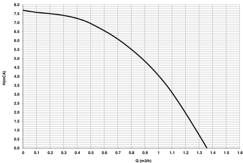
fig. 58 - Prevalenza residua disponibile all'impianto
