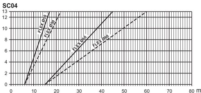
fig. 23 - Grafico per scelta parametro camino
