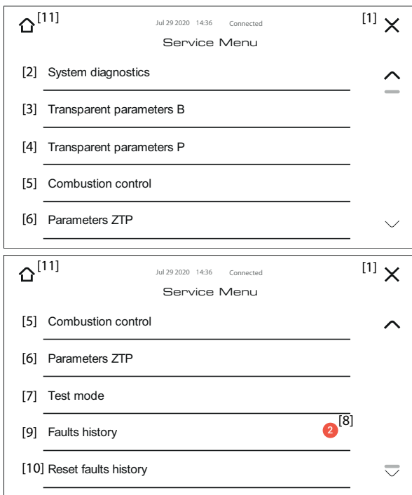
fig. 35- Service Menù
