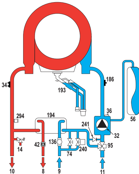
fig. 55- Circuito hidráulico
