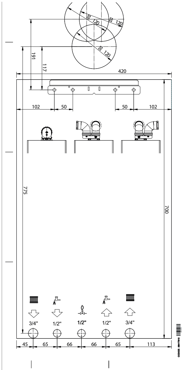
fig. 53- Plantilla de papel
