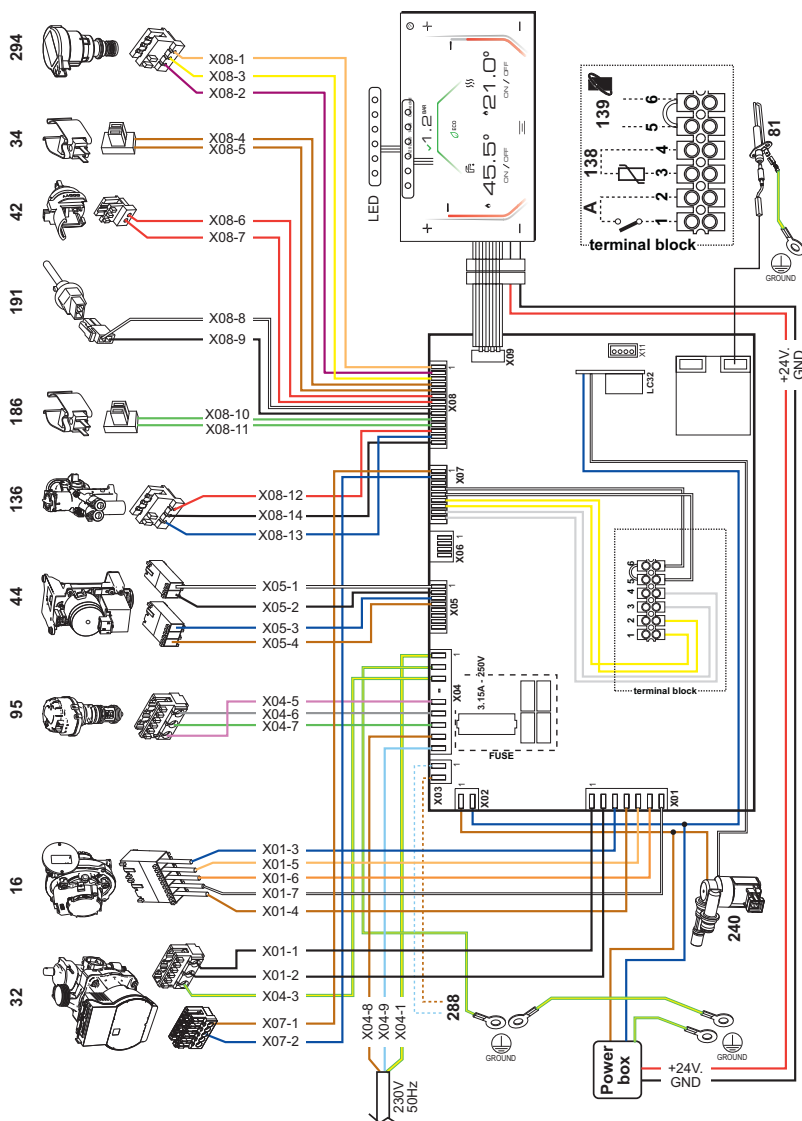
fig. 58- Schema electrică
