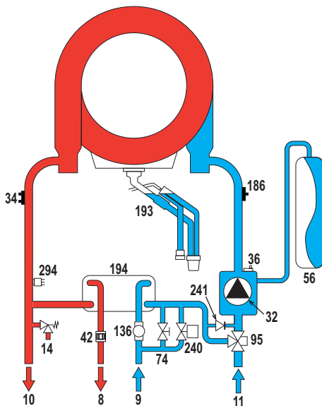
fig. 55- Circuitul hidraulic
