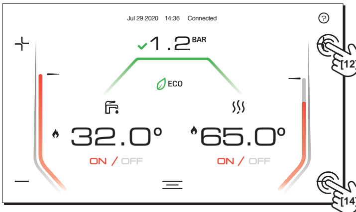
fig. 7- Regulación calefacción
