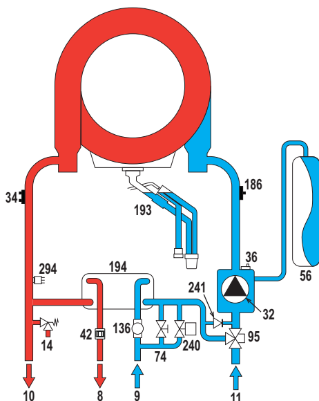
fig. 56 - Circuito idraulico
