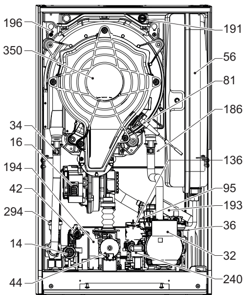
fig. 54- Vedere generală
