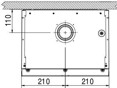
fig. 49- Vista superior
