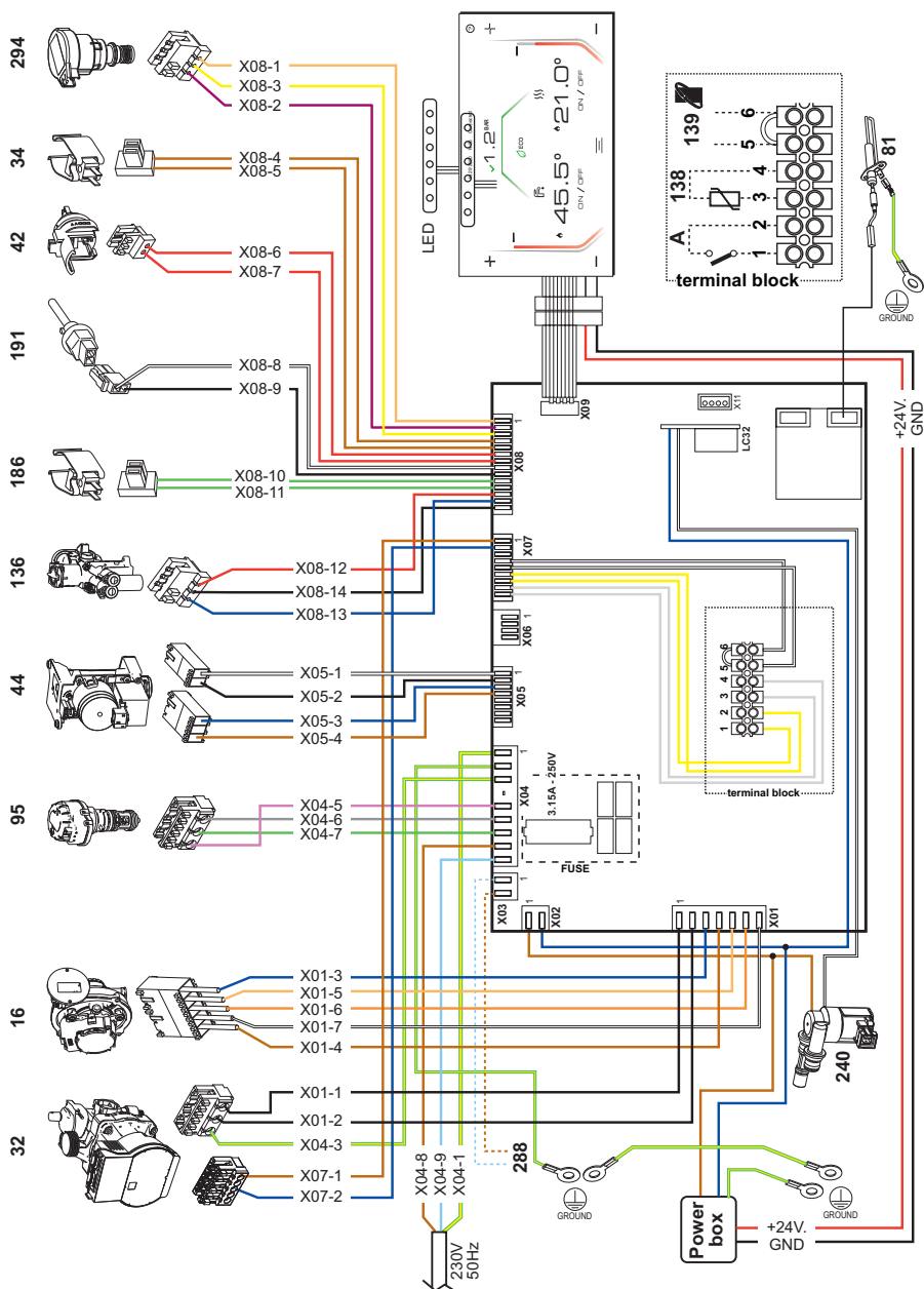
fig. 59 - Schema elettrico
