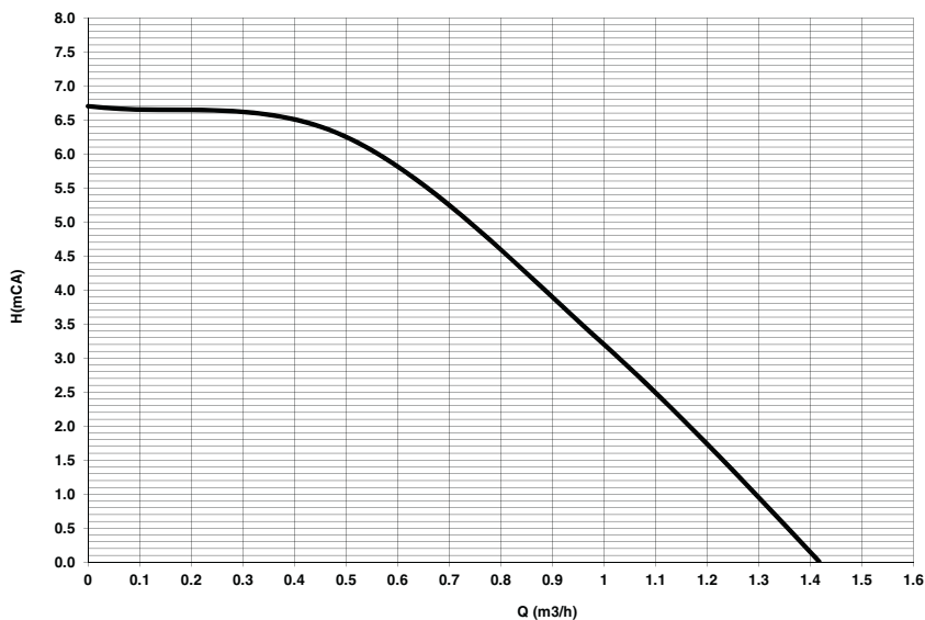
fig. 57 - Prevalenza residua disponibile all'impianto
