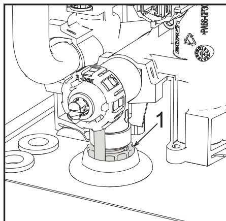
fig. 10 - Valvola di sicurezza con rubinetto di scarico
