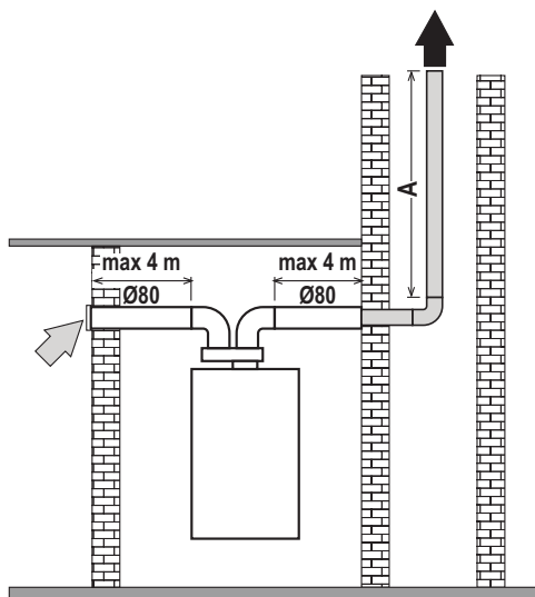
fig. 22- Schemă numai pentru tuburi flexibile
