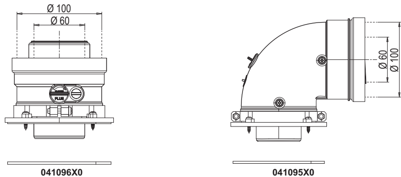
fig. 15- Accesorios iniciales para conductos coaxiales
