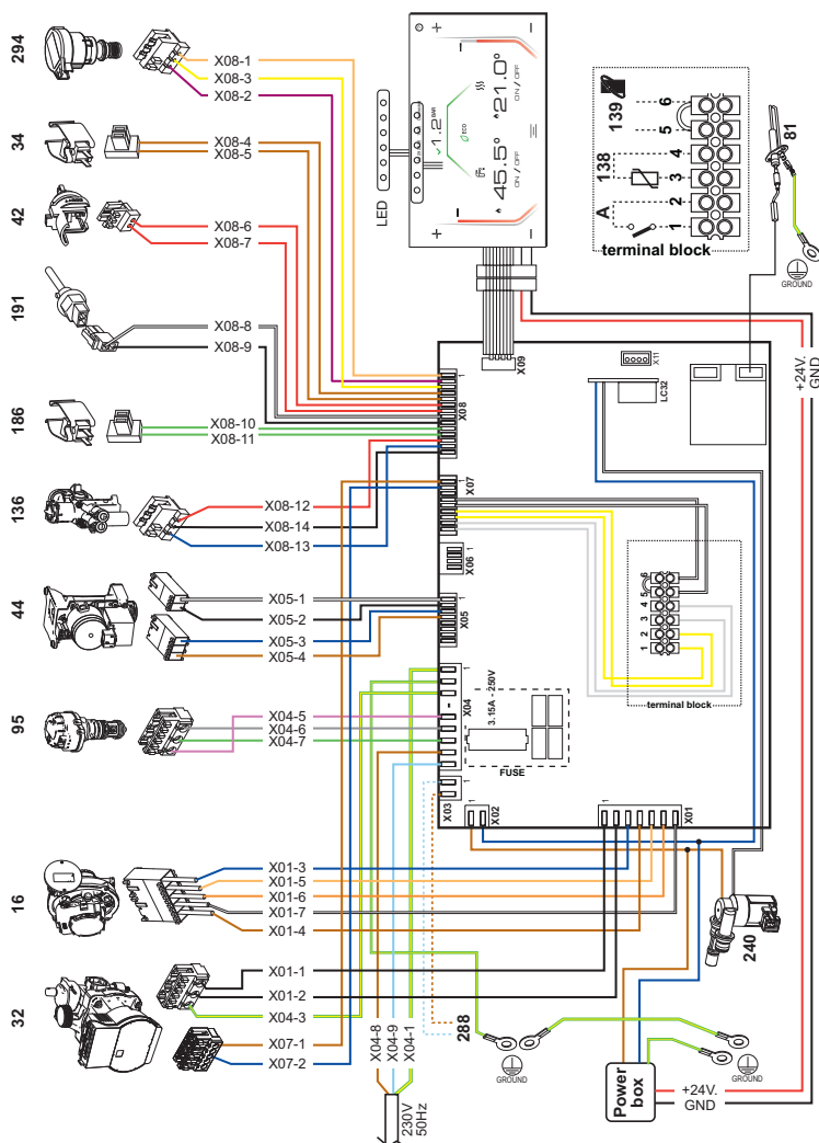
fig. 58- Esquema eléctrico
