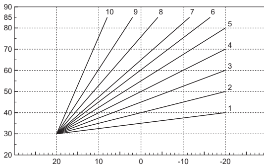
fig. 37- Curvas de compensación
