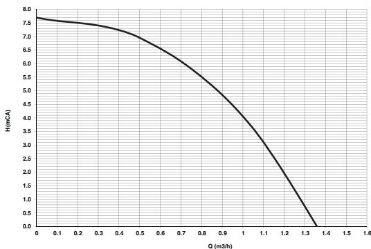
fig. 57- Carga hidrostática residual disponible en la instalación
