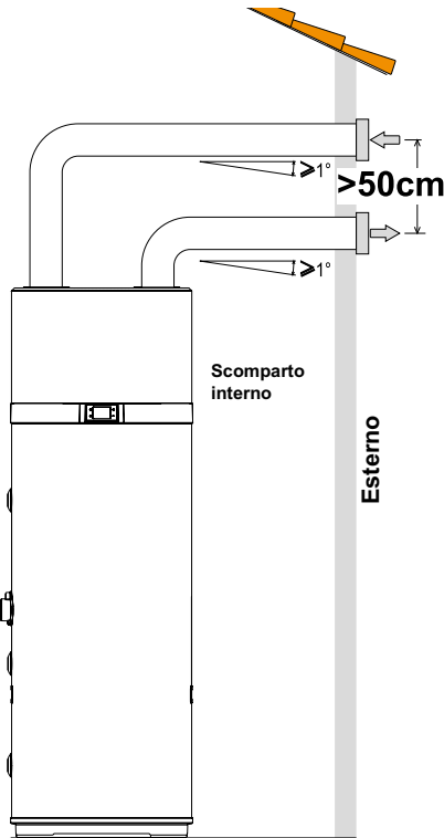
fig. 53- Esempio di collegamento di uscita aria
