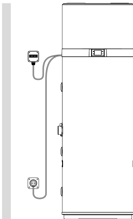
fig. 70- Esempio di collegamento a distanza
