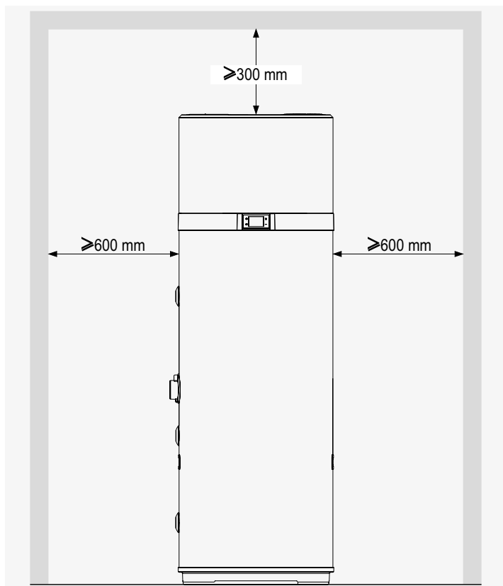
fig. 48 - Spazi minimi
